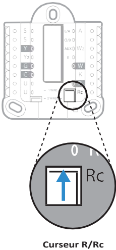
Système de montage UWP
