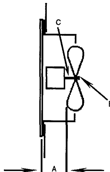
FIGURE 10 FAN BLADE
