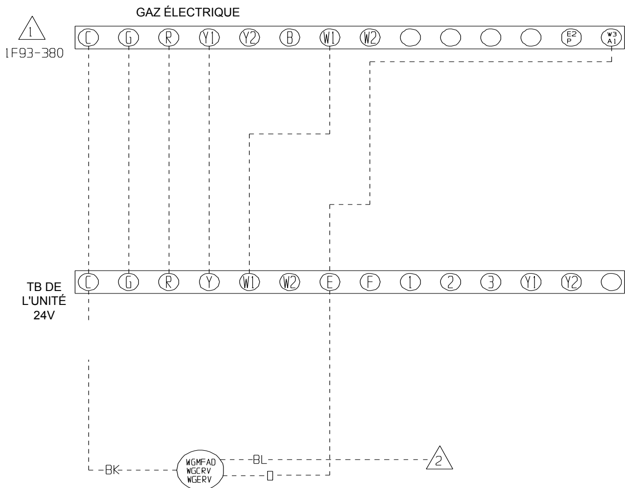
FIGURE 11 FONCTIONNEMENT DE L'APPAREIL AVEC LE WGERV INSTALLÉ
