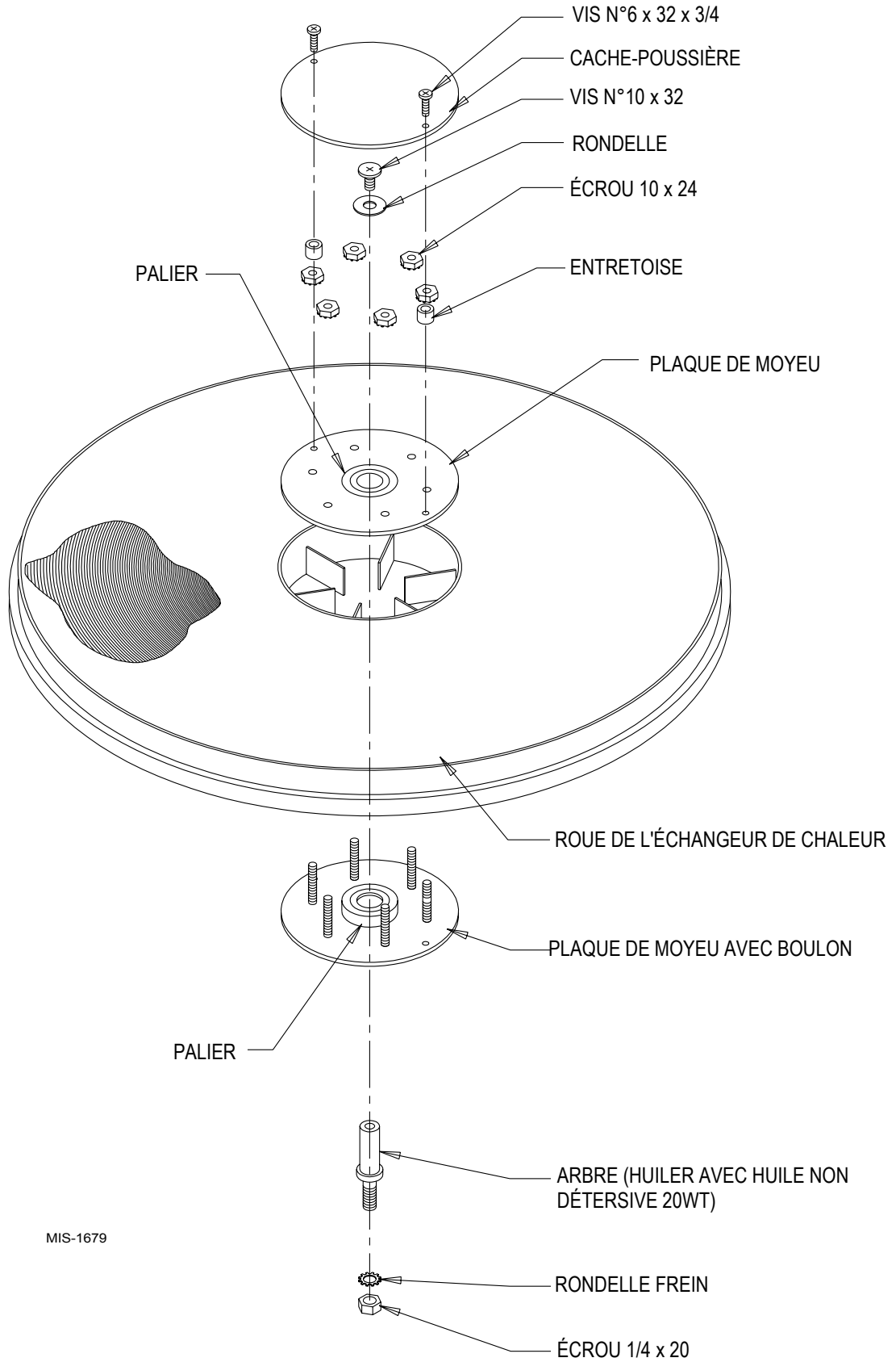
FIGURE 13 MOYEU AVEC PALIER À COUSSINET - DOUILLE
