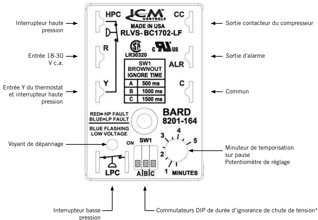
FIGURE 22 Module de commande du compresseur 8201-164
