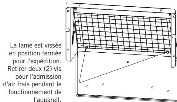
FIGURE 11 Registre d'air frais
