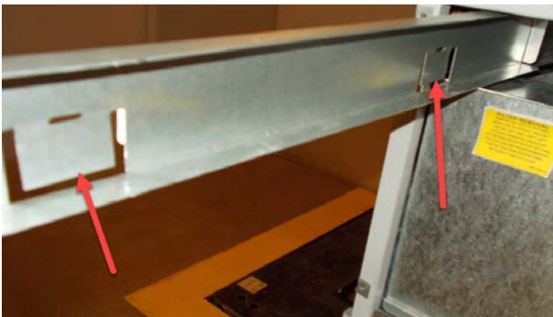
FIGURE 5 Pliage vers le bas des languettes du filtre
