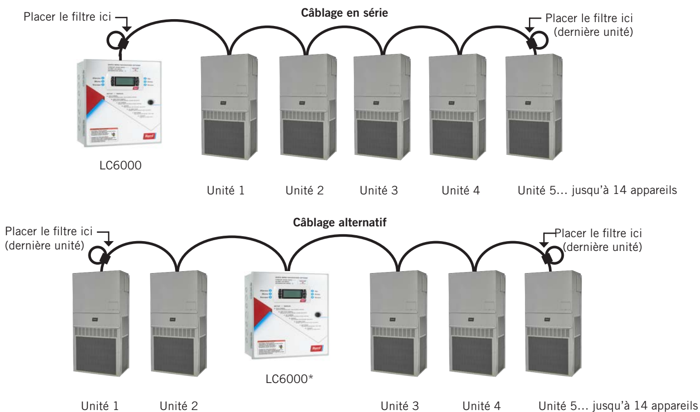
FIGURE 19 Positionnement des filtres de fil de communication (liaison en série ou alternative)
