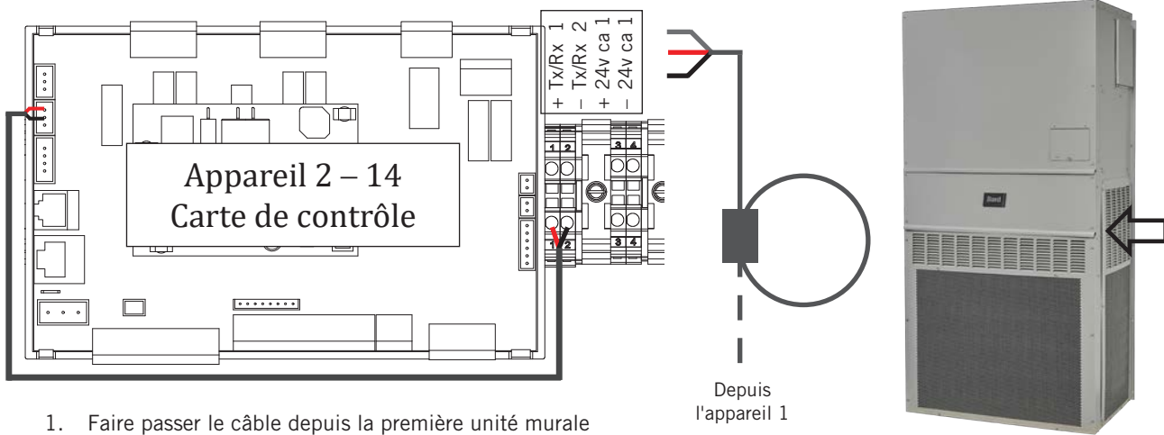
FIGURE 22 Câblage de communication : Terminaison au niveau des appareils murales supplémentaires
