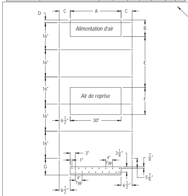
Ouverture murale et emplacement des ouvertures
