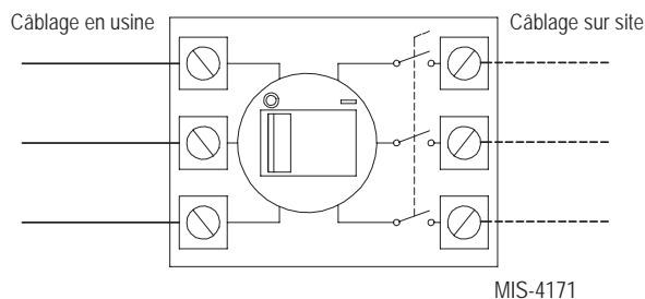
FIGURE 9 Points de connexion du câblage d'alimentation secteur
