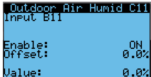
FIGURE 40 Activation/désactivation de la sonde d'humidité d'air extérieur
