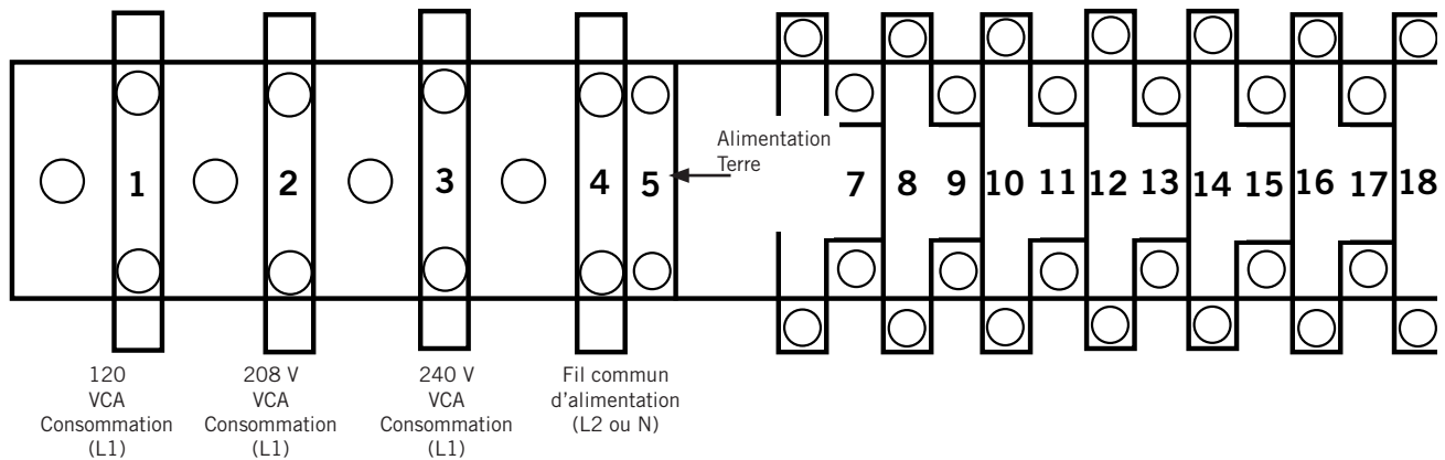
FIGURE 23 Installation du circuit du contrôleur LC6000
