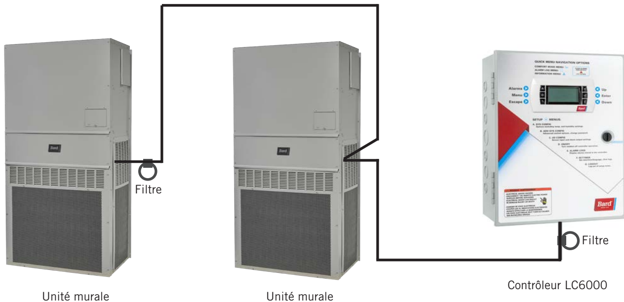
FIGURE 17 Câblage de communication (liaison série)
