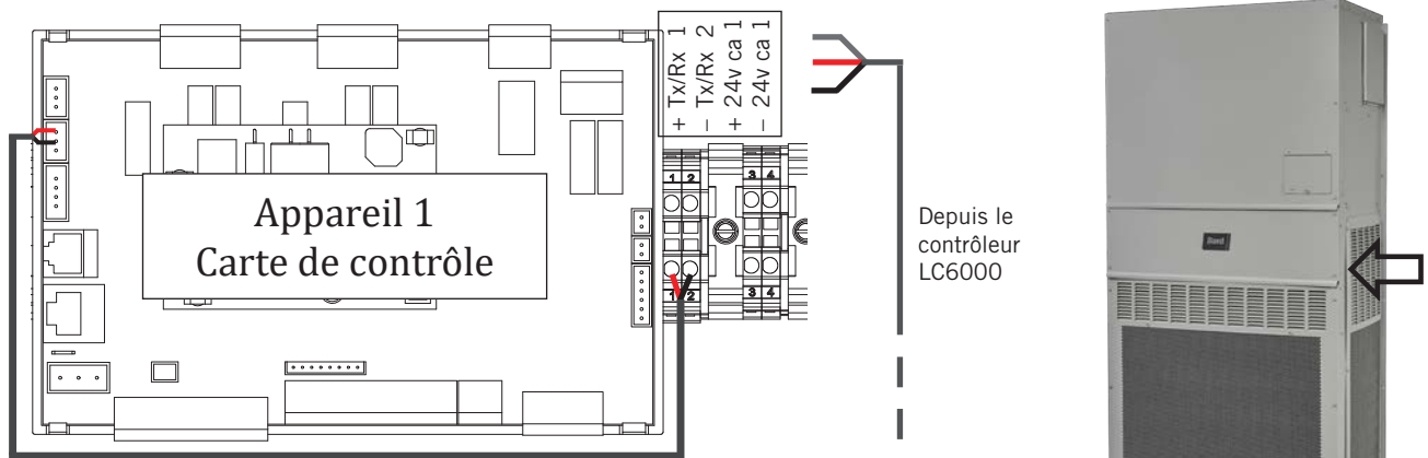
FIGURE 21 Câblage de communication : Terminaison au niveau de la première unité murale
