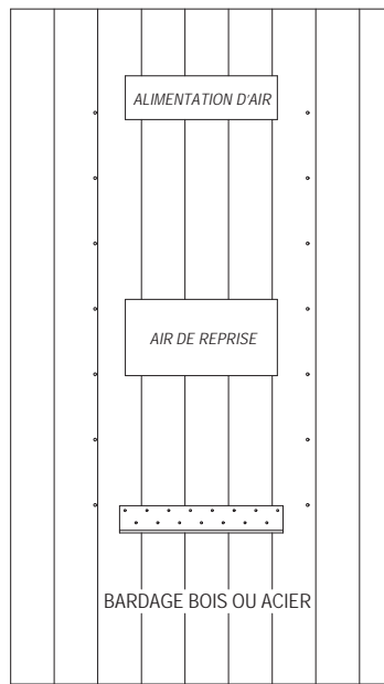
INSTALLATION SUR OSSATURE BOIS
