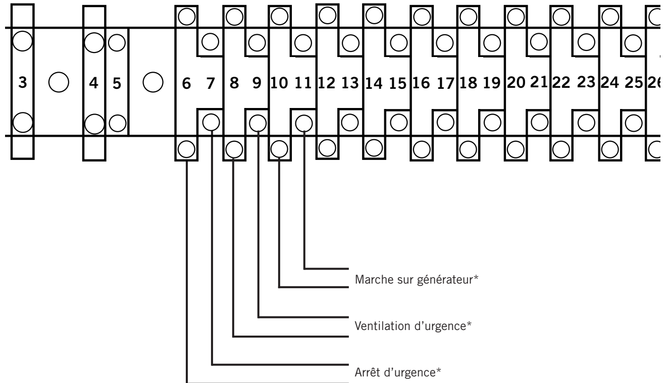
FIGURE 16 Série LC6000-200 – connexion de l'arrêt d'urgence, de la ventilation d'urgence et de la marche sur générateur (le cas échéant)
