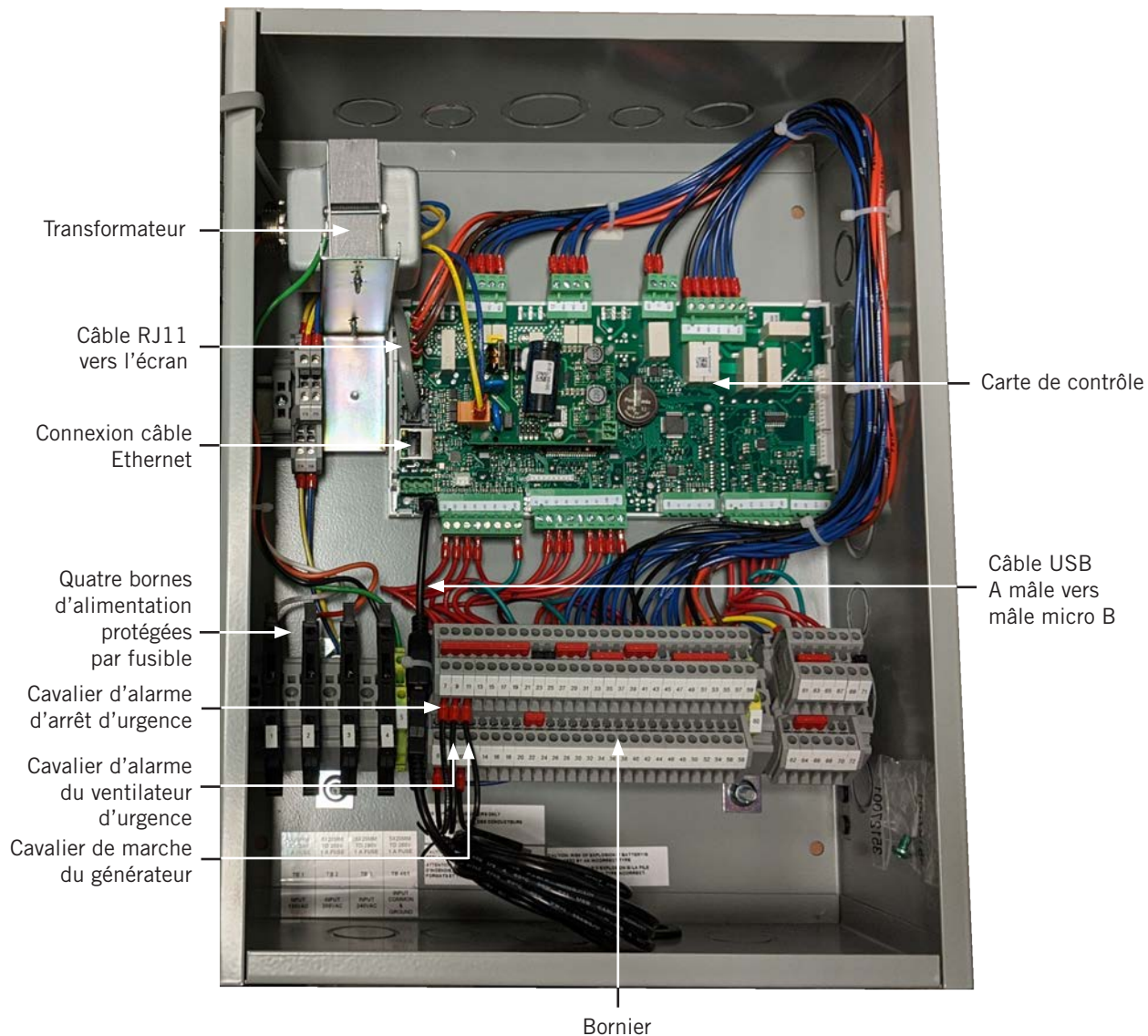
FIGURE 11 Emplacement des composants du LC6000-200
