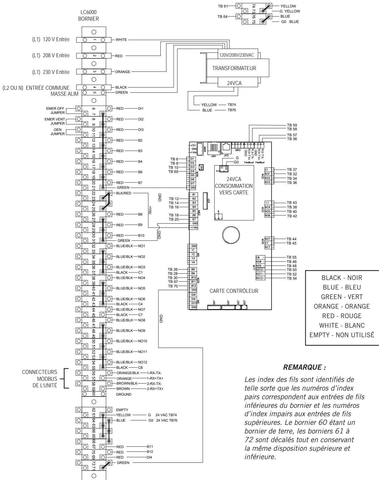
FIGURE 25 Schéma de câblage du LC6000-200
