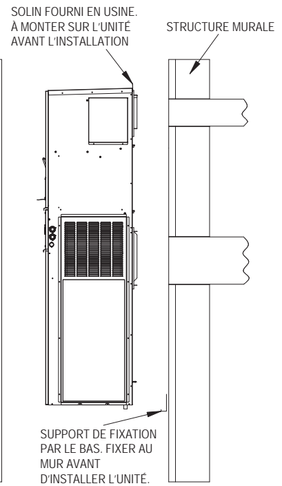
VUE LATÉRALE
