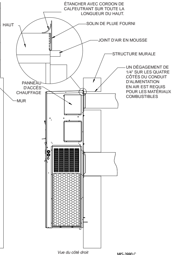
Vue du côté droit
