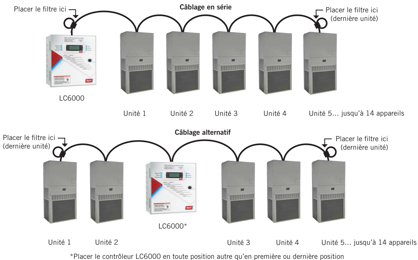
FIGURE 19 Positionnement des filtres de fil de communication (liaison en série ou alternative)
