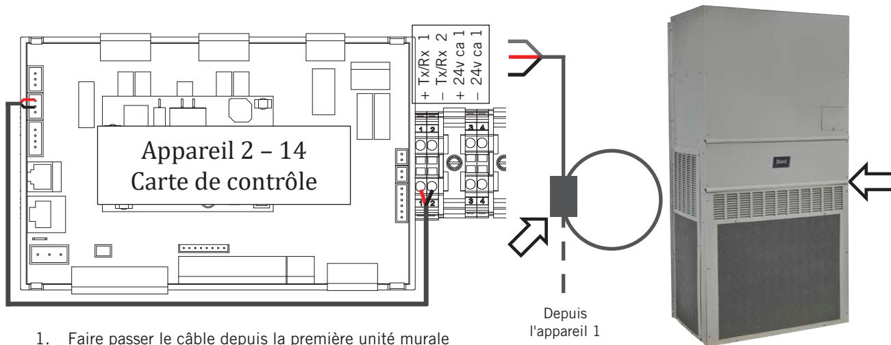
FIGURE 22 Câblage de communication : Terminaison au niveau des appareils muraux supplémentaires
