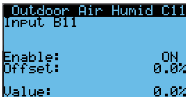
FIGURE 40 Activation/désactivation de la sonde d'humidité d'air extérieur
