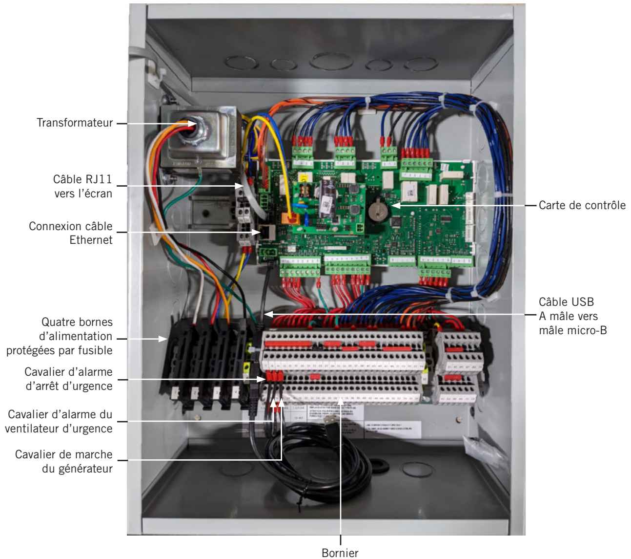
FIGURE 11 Emplacement des composants du LC6000-200
