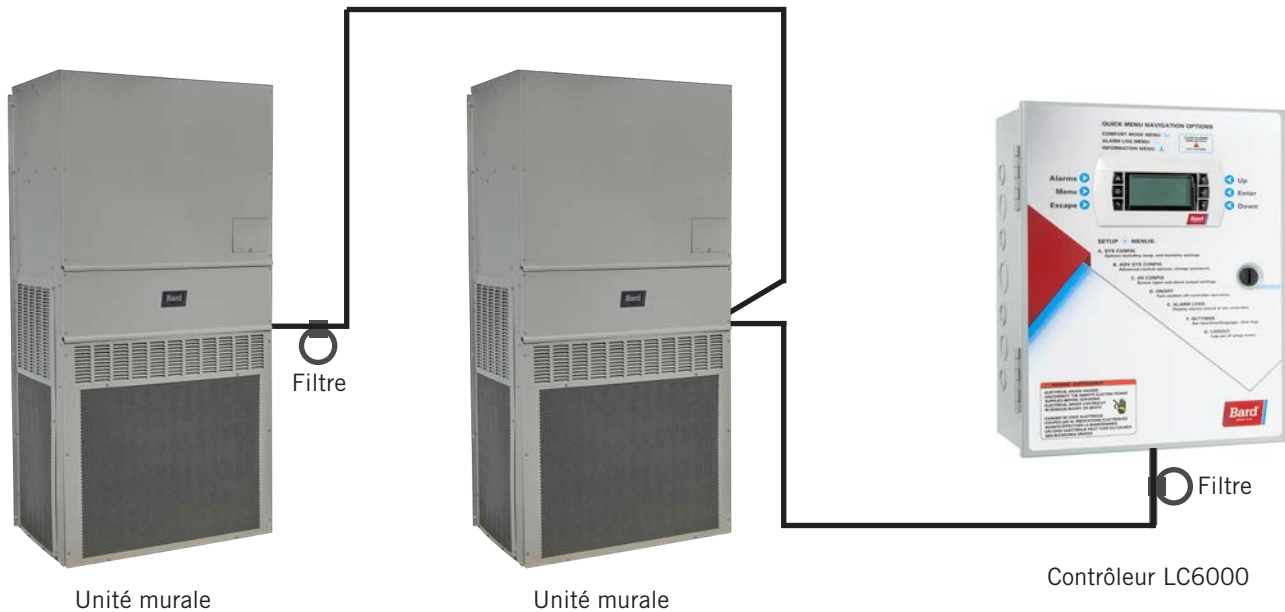
FIGURE 17 Câblage de communication (liaison série)
