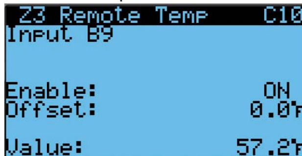
FIGURE 39 Activation/désactivation de la sonde distante de température zone 3
