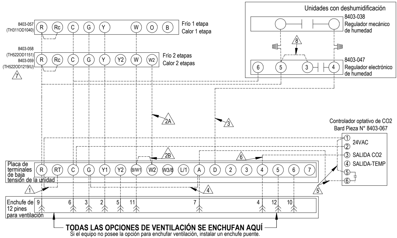
FIGURA 9 Conexiones de termostato no programable
