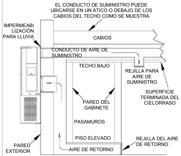
INSTALACIÓN DEL GABINETE
