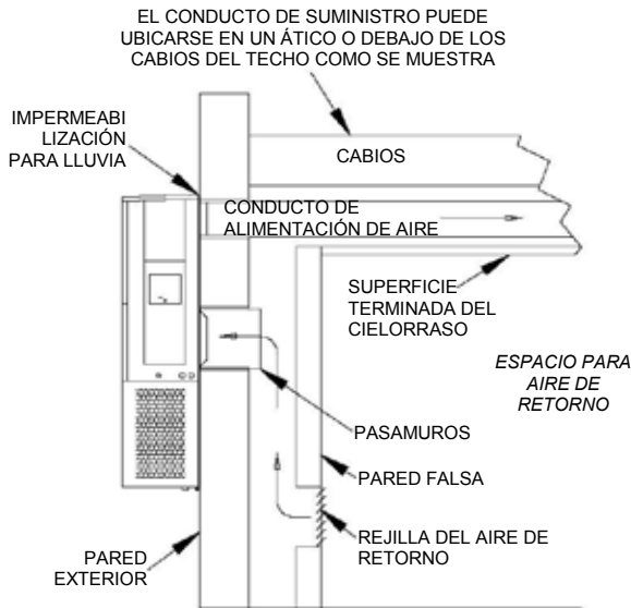
INSTALACIÓN DE LA PARED FALSA
