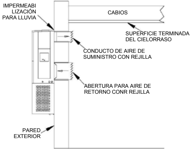
FLUJO DE AIRE LIBRE SIN CONDUCTO
