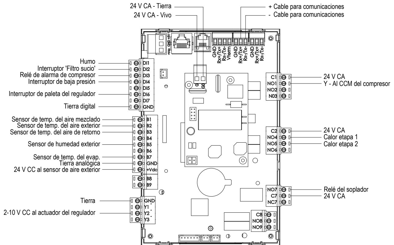
FIGURA 21 Placa de control de la unidad de montaje en la pared
