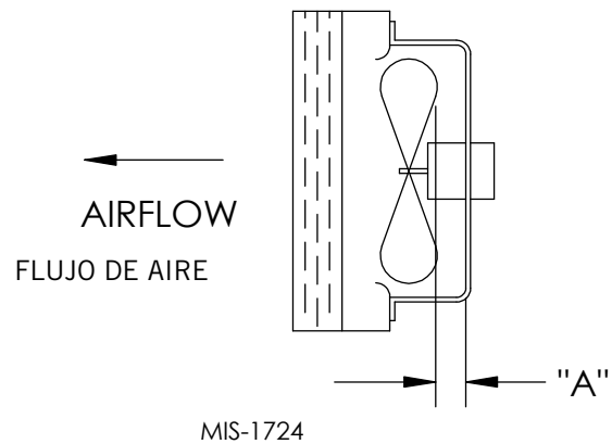
FIGURA 22 Ajuste de las paletas del ventilador
