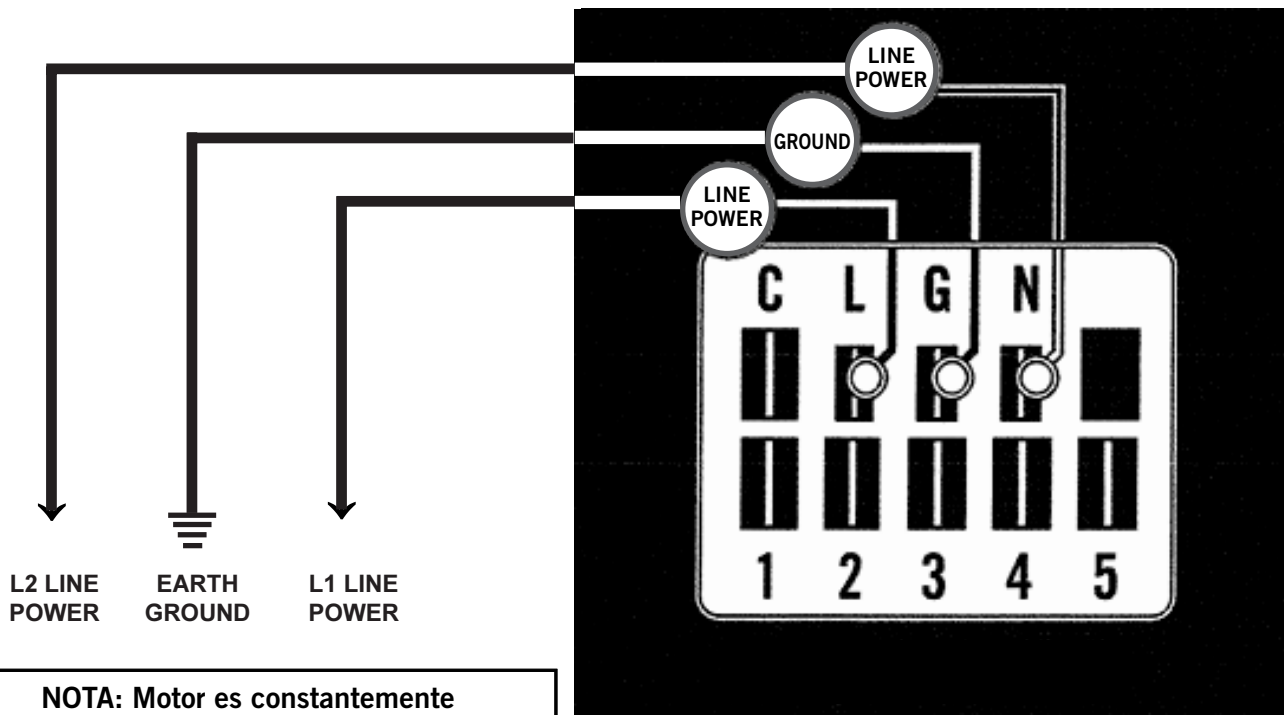
FIGURA 27 Conexiones del motor
