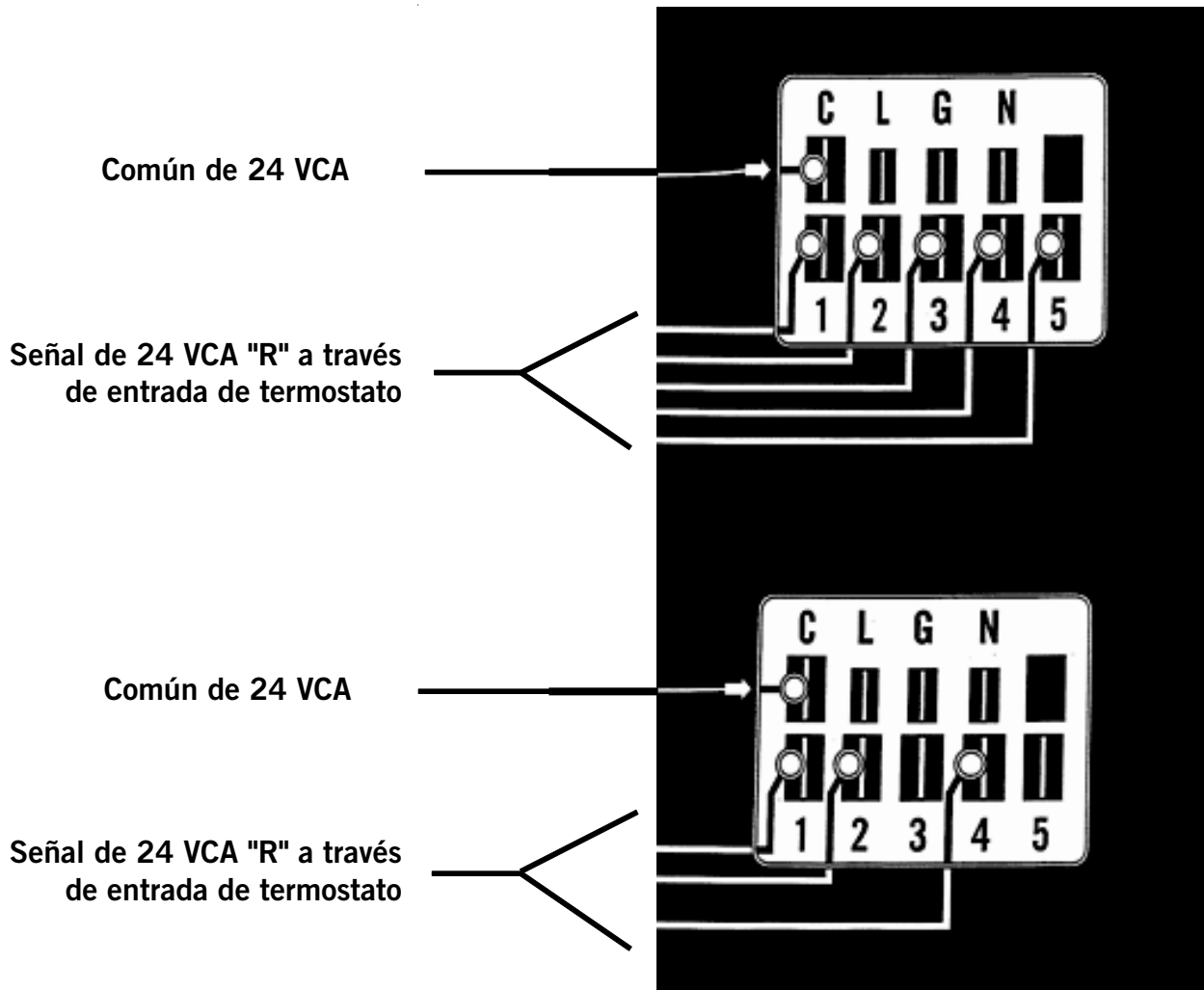
FIGURA 28 Conexiones del motor
