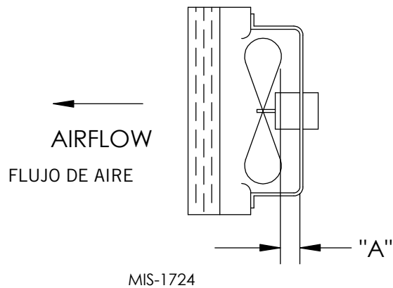
FIGURA 26 Ajuste de las paletas del ventilador
