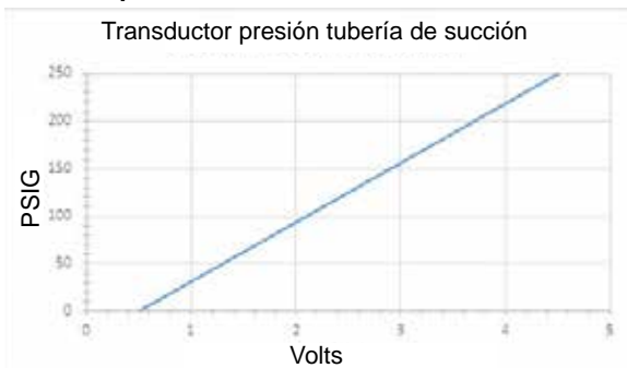
FIGURA 20 Voltaje en función de la presión: Transductor de presión de la tubería de succión
