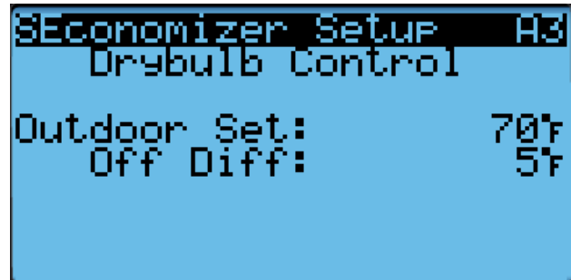
FIGURA 44 Configuración del economizador – Control de Temp./Hum.
