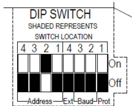
FIGURE 66 Compruebe la posición del interruptor DIP
