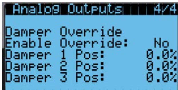
FIGURA 34 Anulación del control automático de la compuerta
