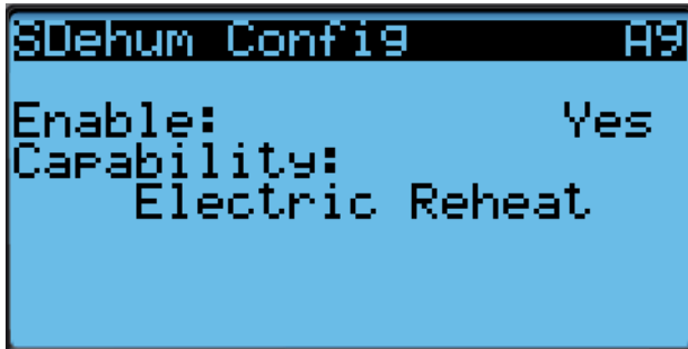
FIGURA 49 Deshumidificación por calefacción eléctrica
