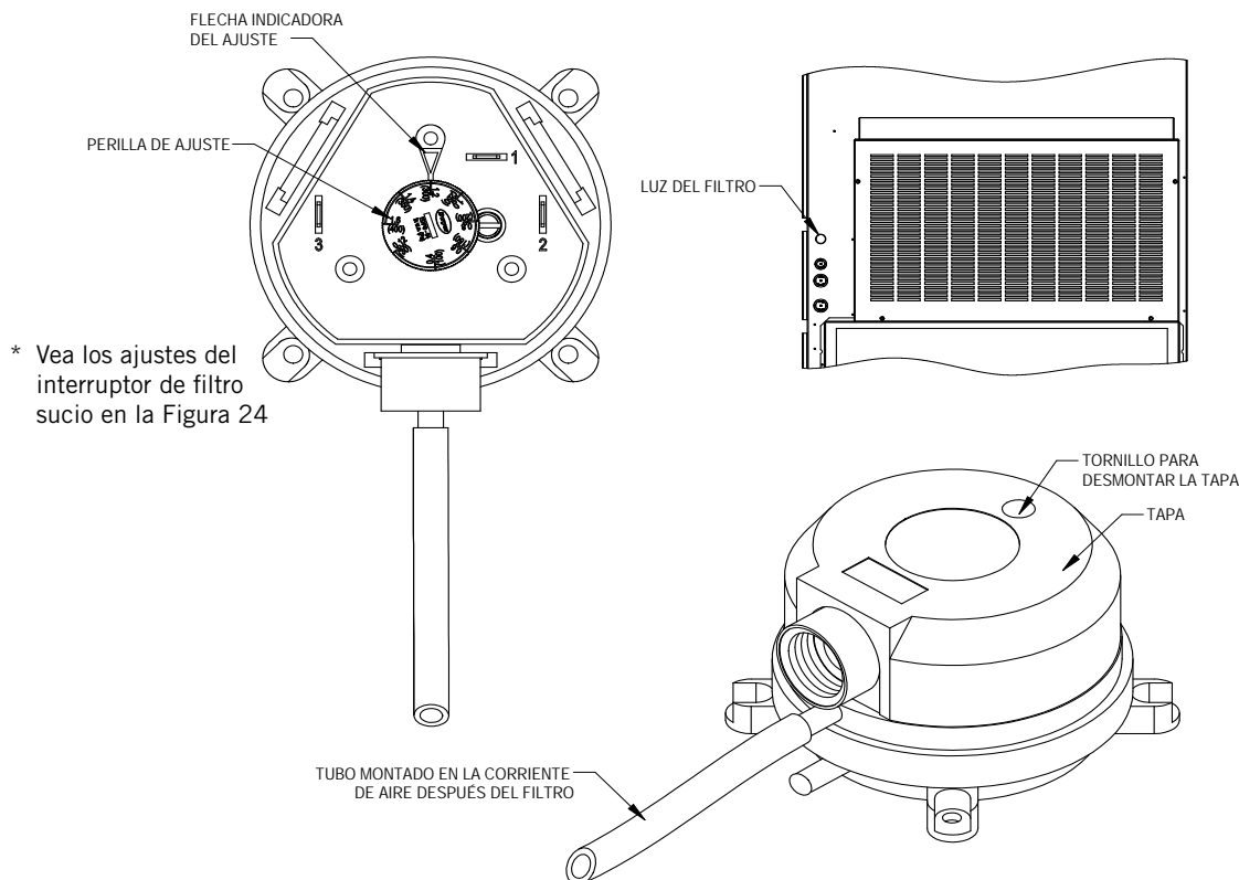
FIGURA 26 Interruptor de filtro sucio y luz indicadora del filtro
