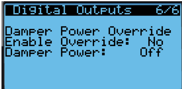
FIGURE 53 Anular la salida del amortiguador
