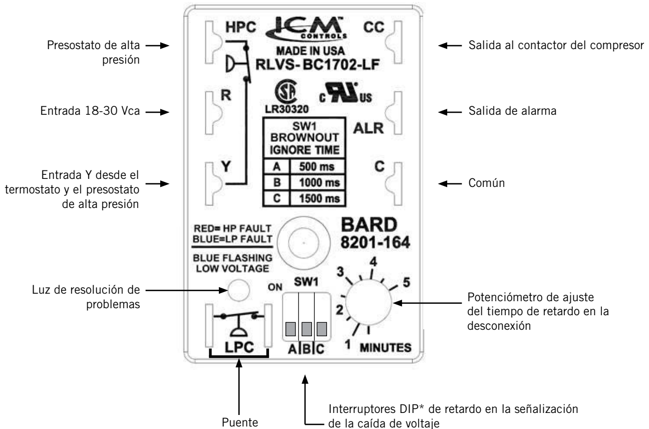
FIGURA 32 Módulo de control del compresor 8201-164
