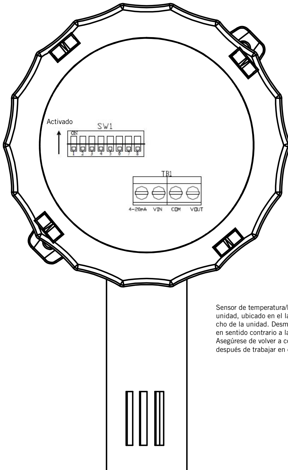
FIGURA 58 Bornes e interruptores DIP del sensor 8301-089
