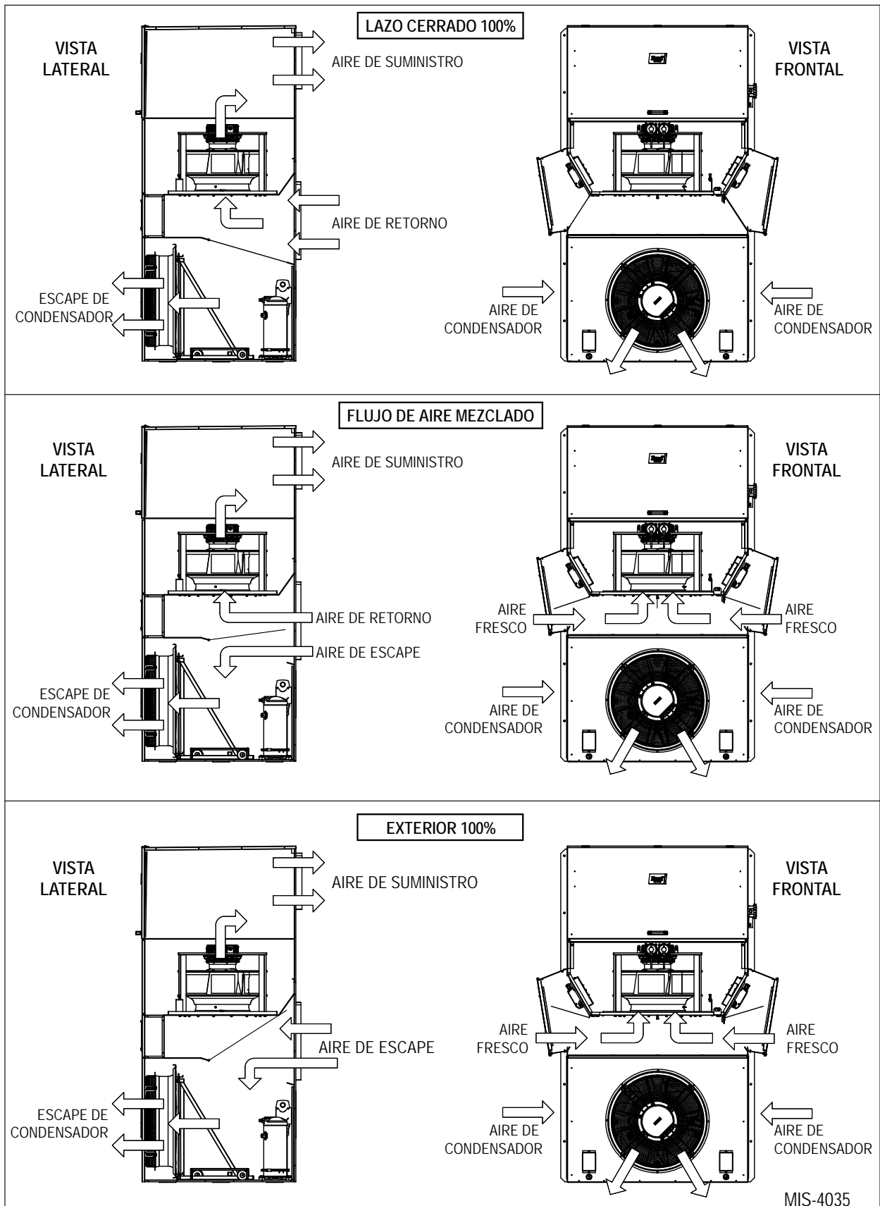
FIGURA 63 Recorridos del flujo de aire de la unidad
