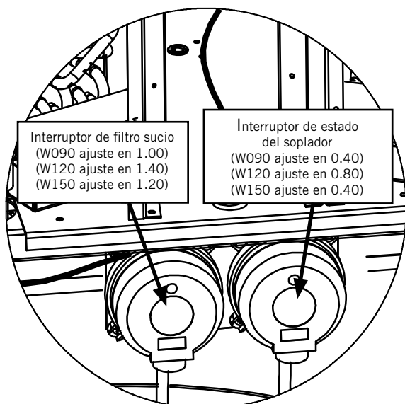
FIGURA 24 Interruptor de filtro sucio e interruptor de estado del soplador
