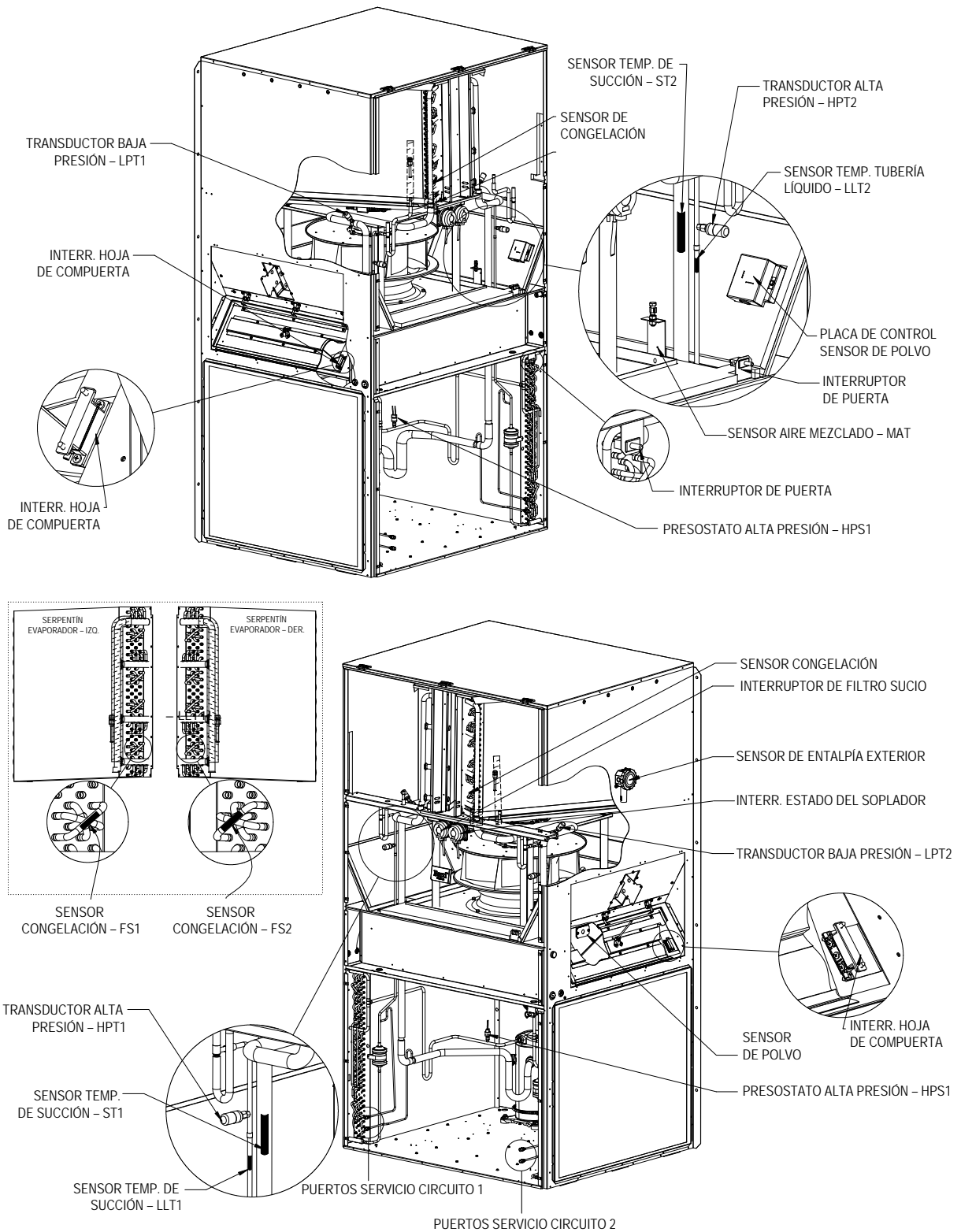
FIGURA 56 Sensores y dispositivos periféricos
