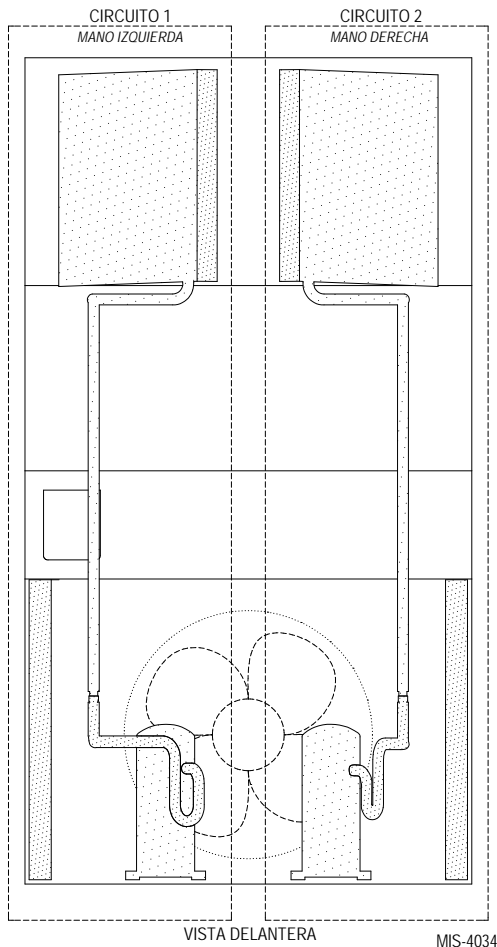
FIGURA 5 Circuitos de enfriamiento de MEGA-TEC
