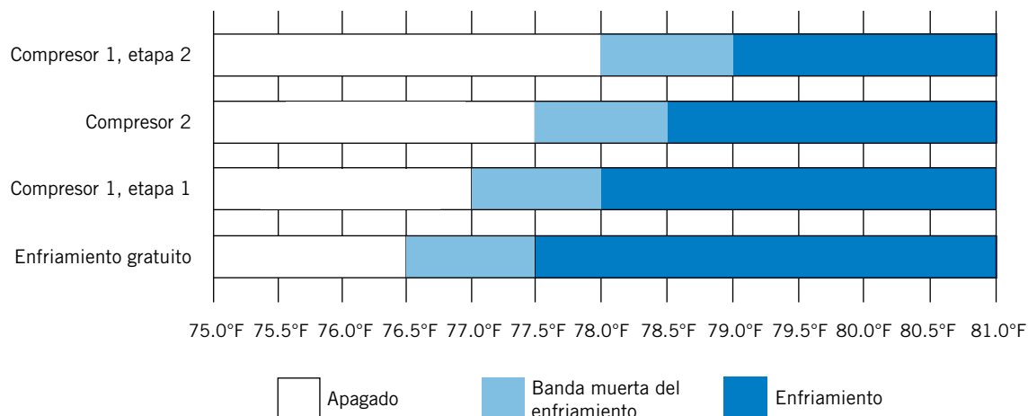
FIGURA 14 Enfriamiento (con economizador)
