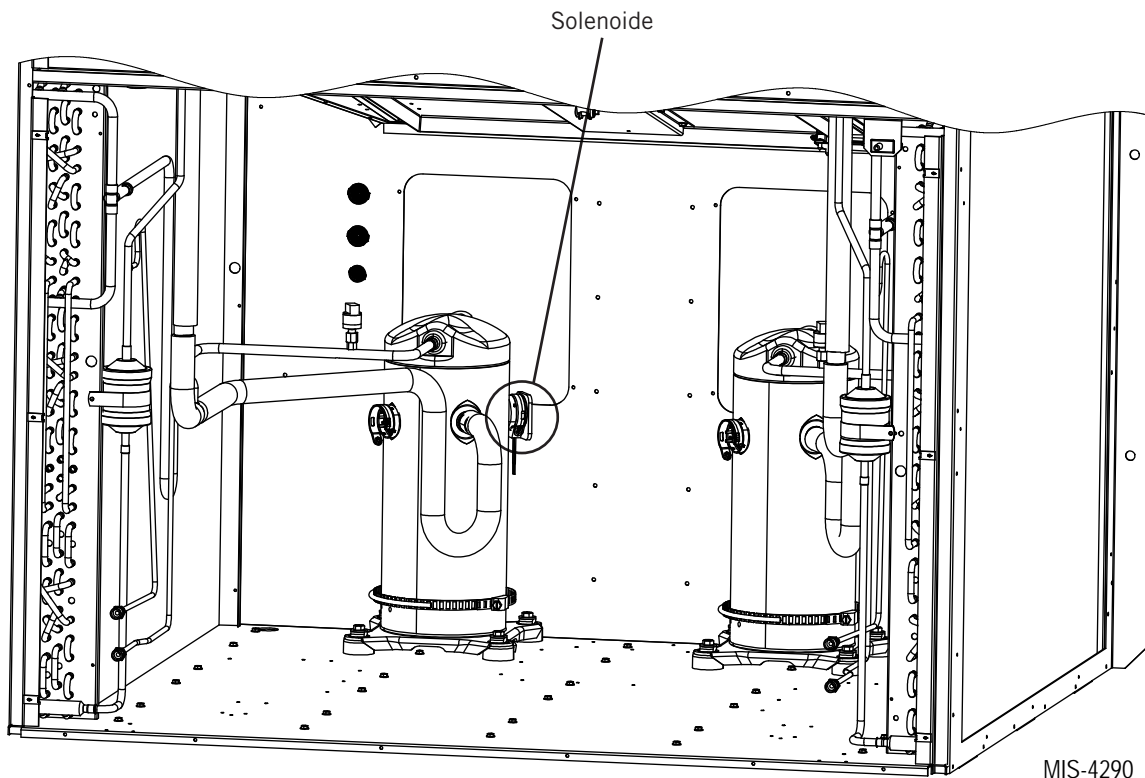
FIGURA 78 Ubicación del solenoide del compresor
