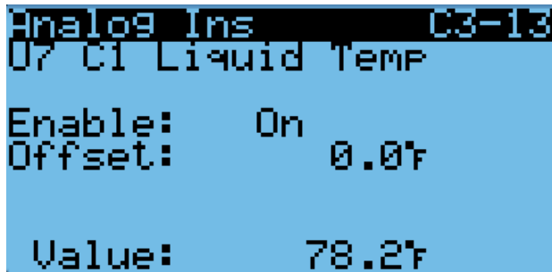
Ajuste de la entrada de temperatura de la tubería de descarga/líquido
