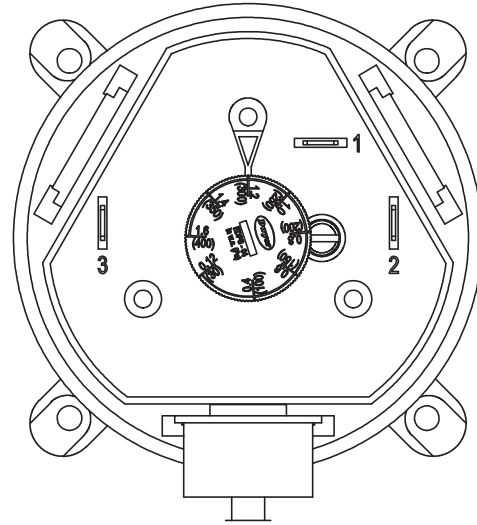
FIGURA 77 Interruptor del diferencial del aire 8301-057
