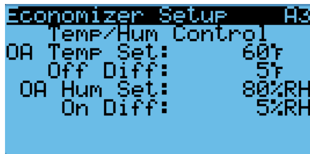
FIGURA 56 Configuración del economizador – Control de Temp./Hum.
