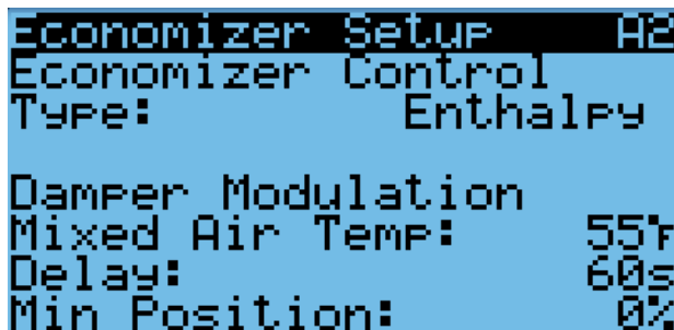
FIGURA 54 Configuración del economizador
