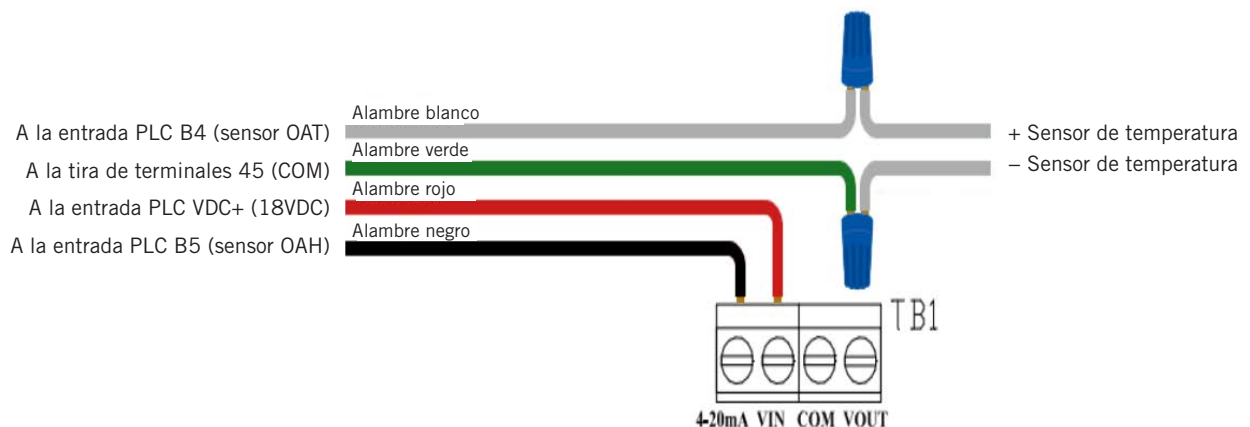
FIGURA 73 Conexiones de terminales de sensor 8301-089
