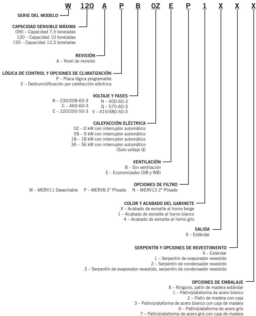
FIGURA 69 Nomenclatura de modelo de la unidad de montaje en pared MEGA-TEC
