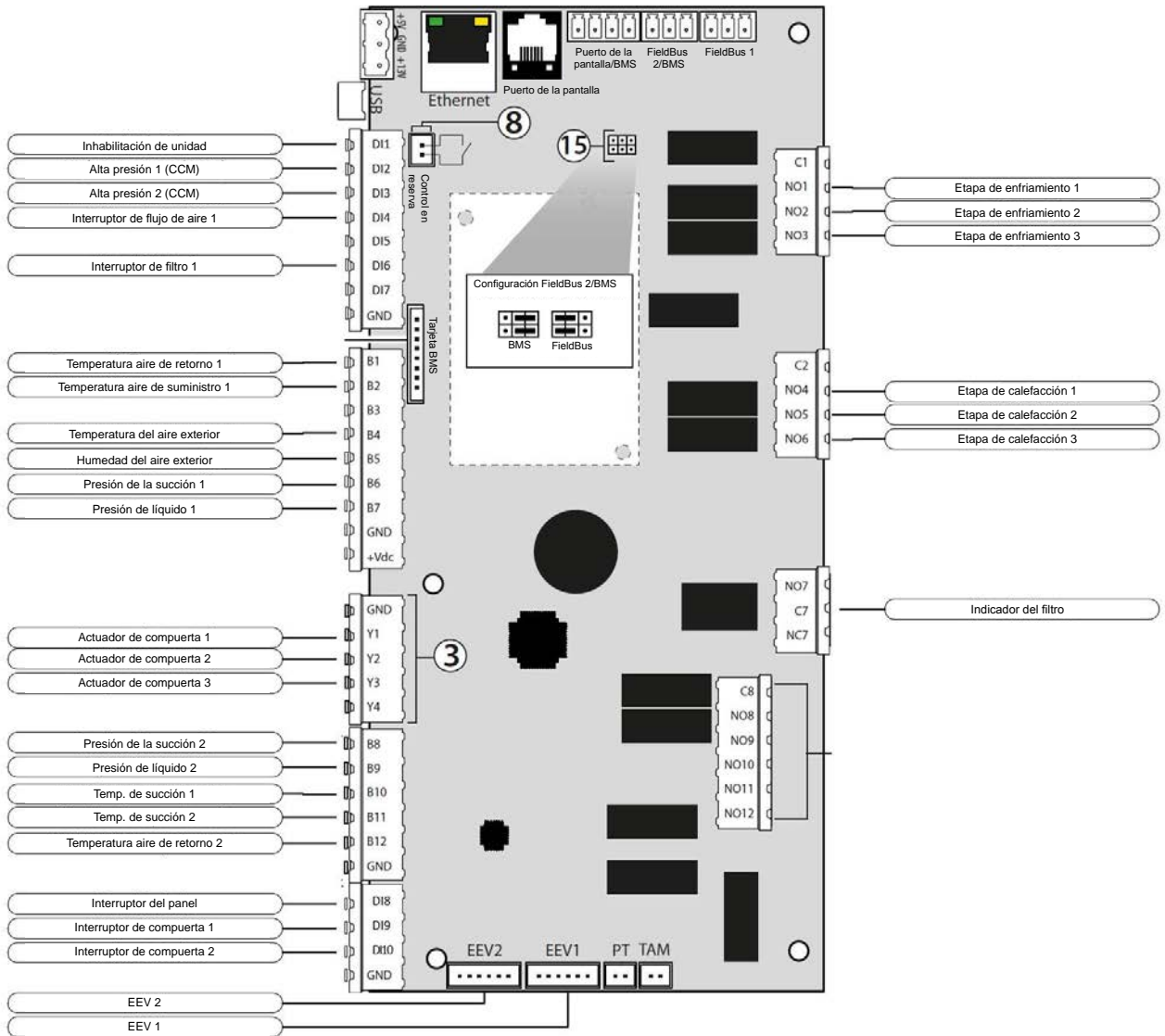
FIGURA 91 Disposición de E/S
