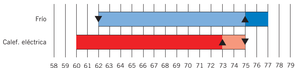
FIGURA 64 Control de la deshumidificación (°F)
