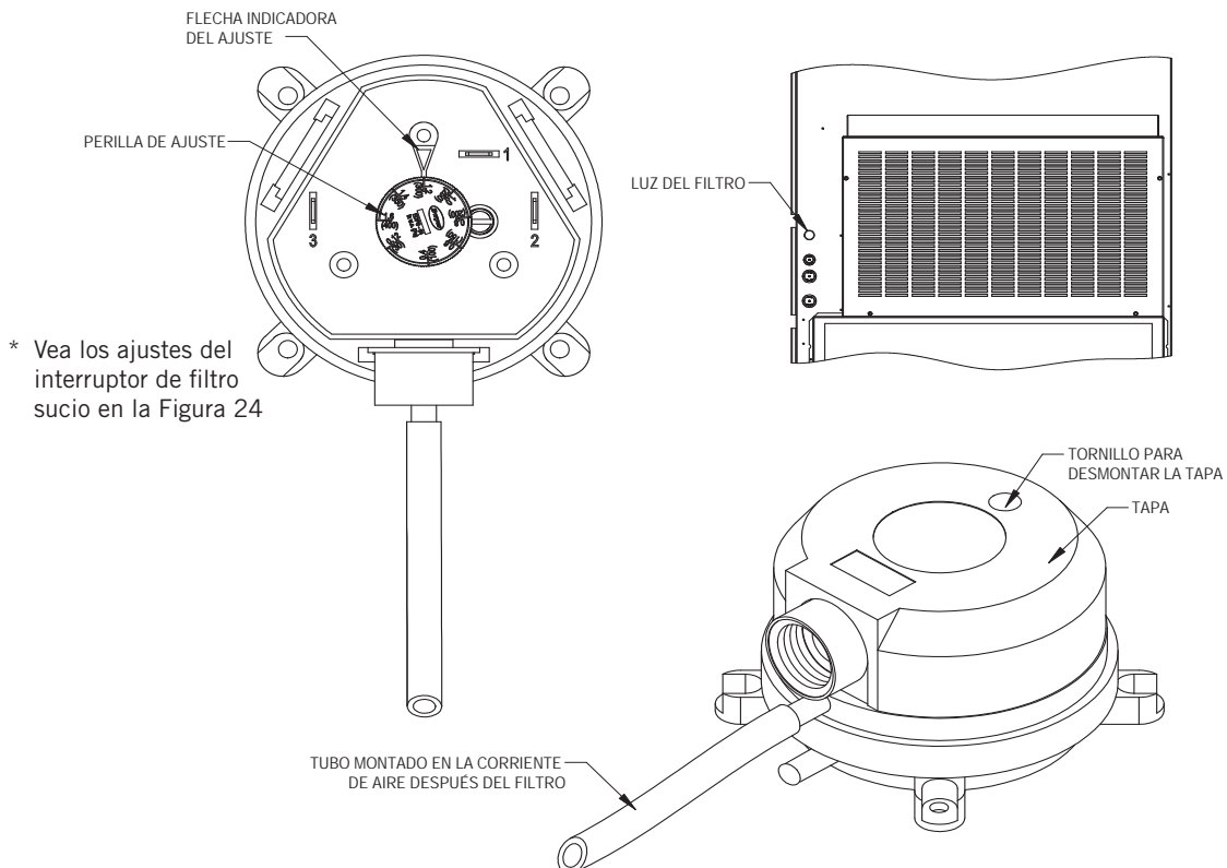
FIGURA 30 Interruptor de filtro sucio y luz indicadora del filtro
