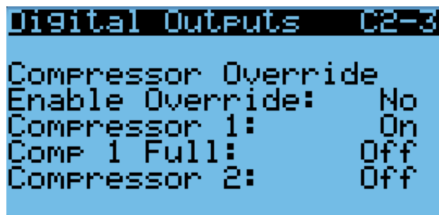
FIGURA 42 Anulación de las salidas del compresor
