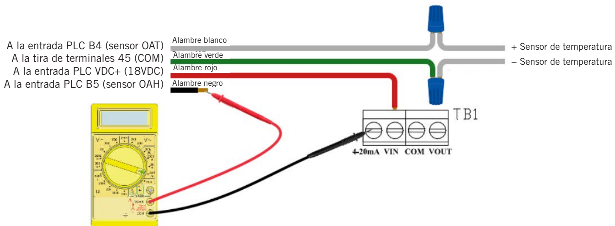
FIGURA 76 Sensor 8301-089: Solución de problemas de la sonda de humedad
