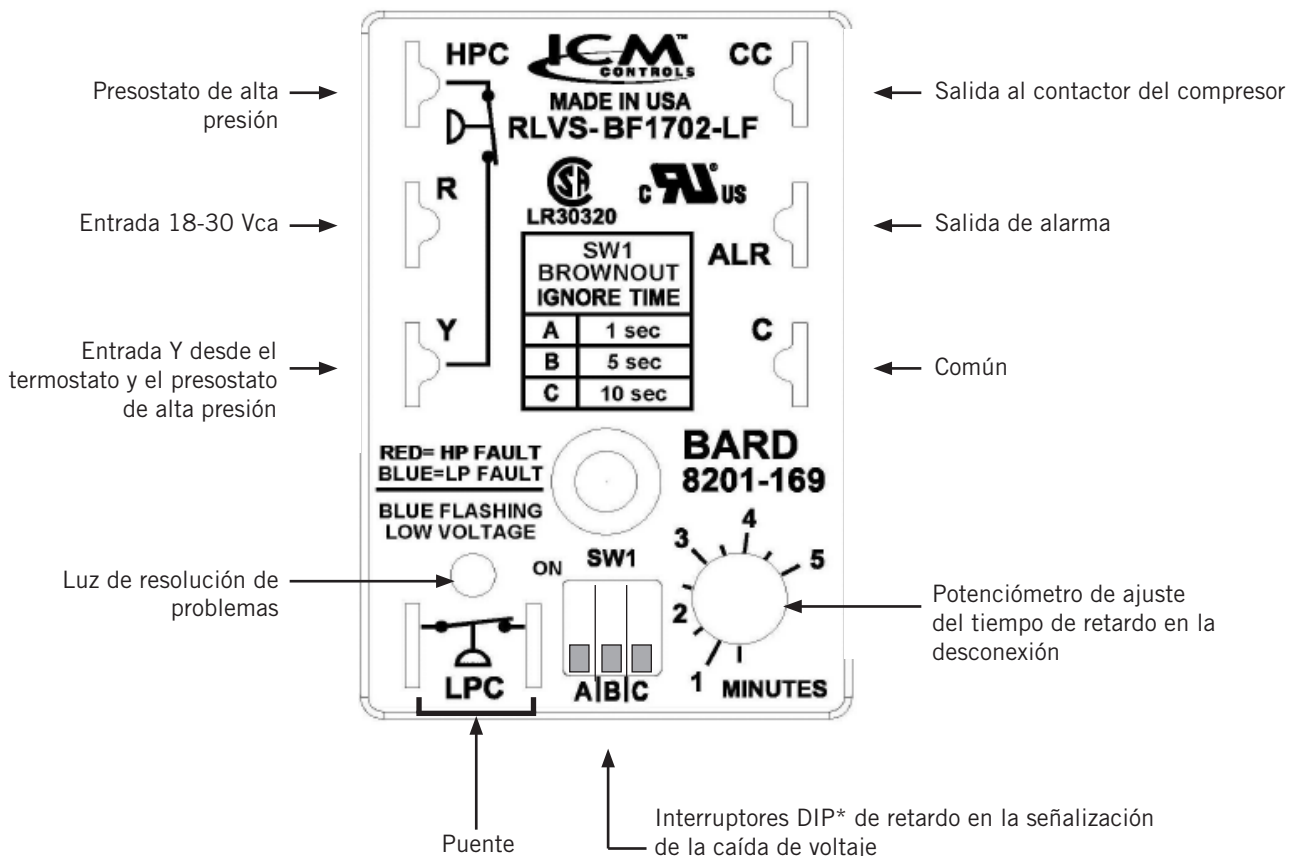
FIGURA 39 Módulo de control del compresor 8201-169
