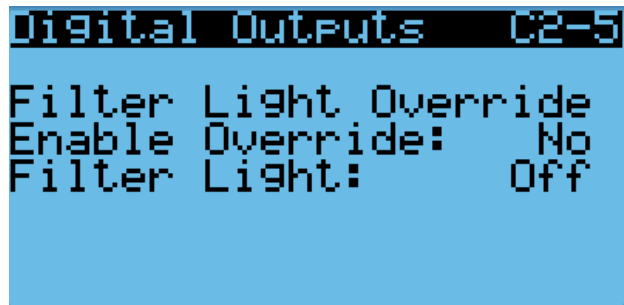
FIGURA 32 Anulación de la salida de luz de filtro
