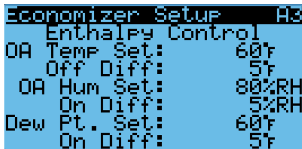
FIGURA 57 Configuración del economizador – Control de entalpía
