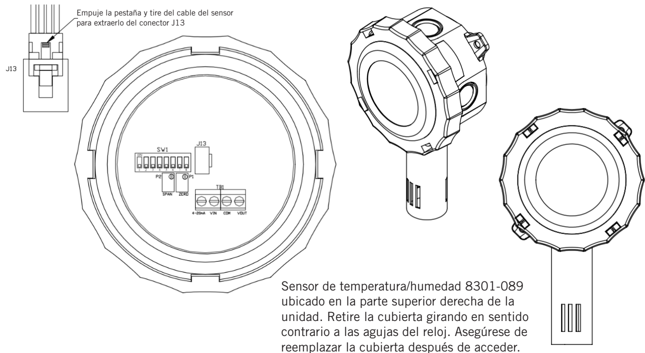
FIGURA 72 Conexiones eléctricas de sensores e interruptores DIP 8301-089
