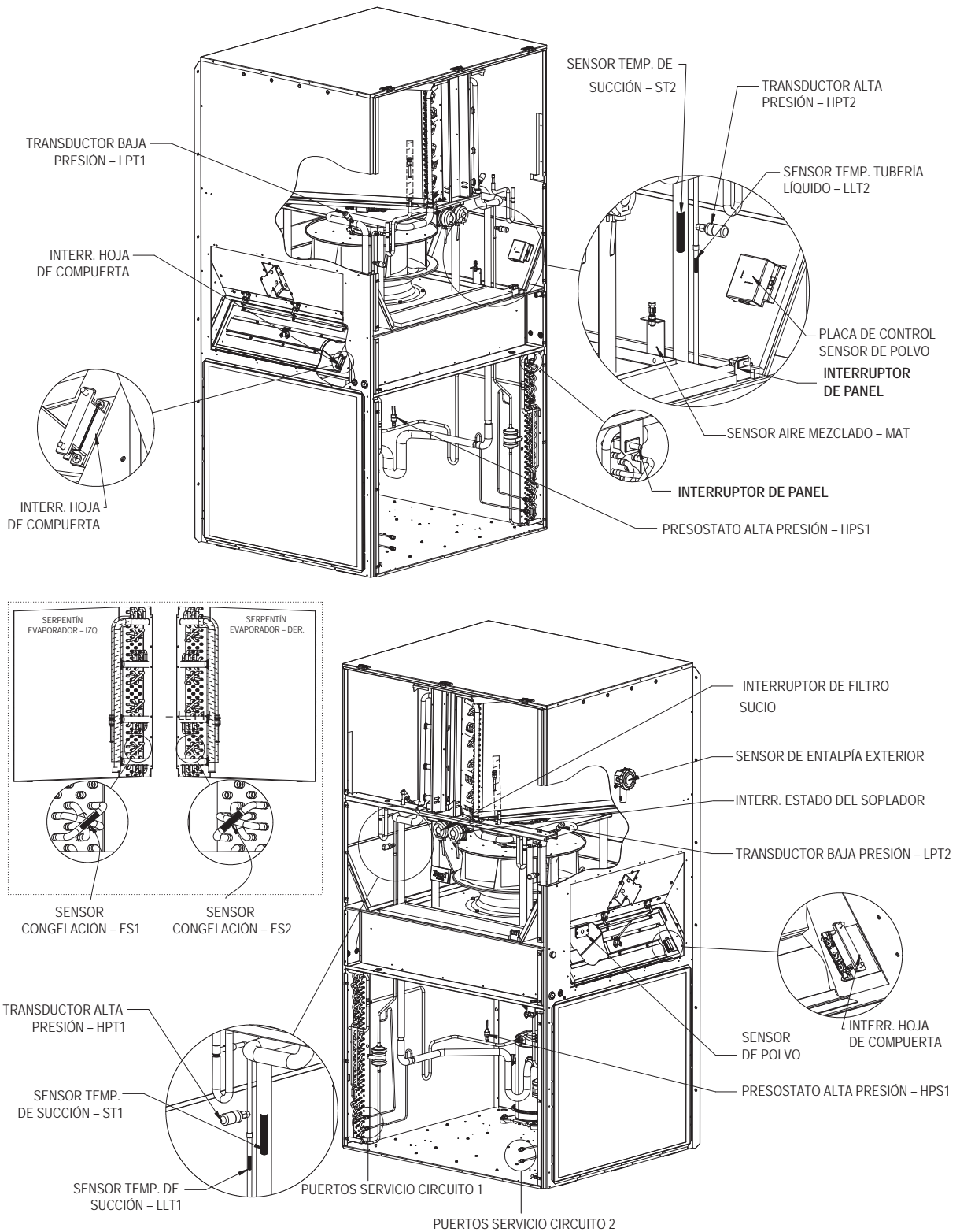
FIGURA 70 Sensores y dispositivos periféricos
