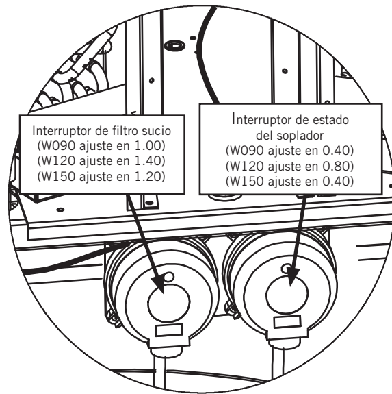
FIGURA 28 Interruptor de filtro sucio e interruptor de estado del soplador
