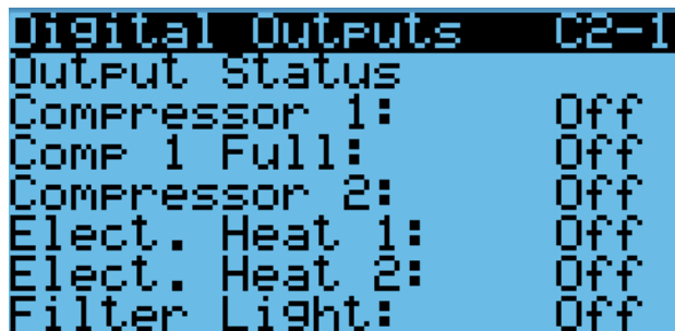
FIGURA 31 Verificación del estado de la luz del filtro
