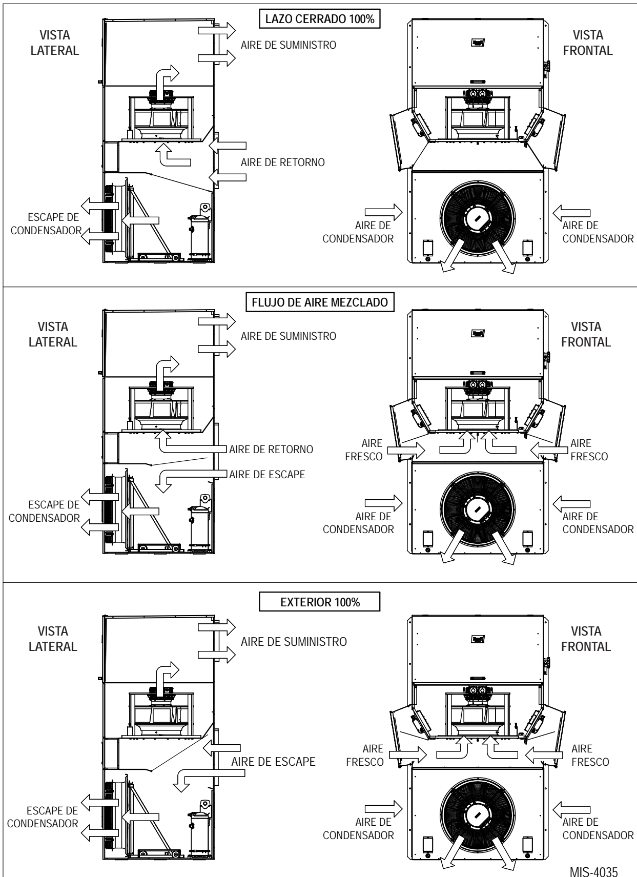
FIGURA 90 Recorridos del flujo de aire de la unidad
