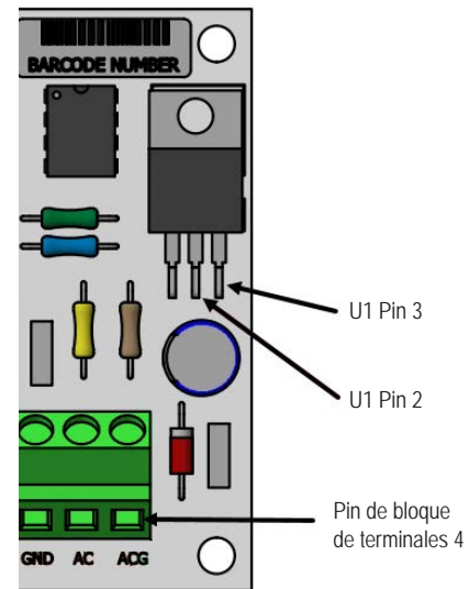
FIGURA 80 Placa de alarma del sensor de polvo 8612-061
