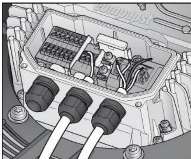
FIGURA 82 Terminales de ventilador
