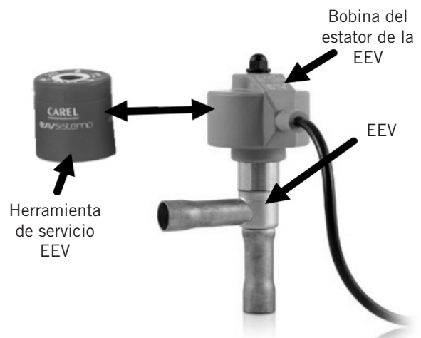
FIGURA 23 Válvula de expansión electrónica (EEV) y herramienta de servicio
