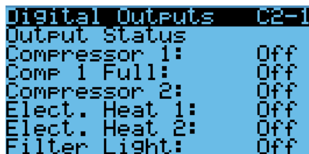
FIGURA 61 Verificación del estado de salida de calor eléctrico
