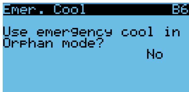
FIGURA 59 Enfriamiento de emergencia – Modo Autónomo
