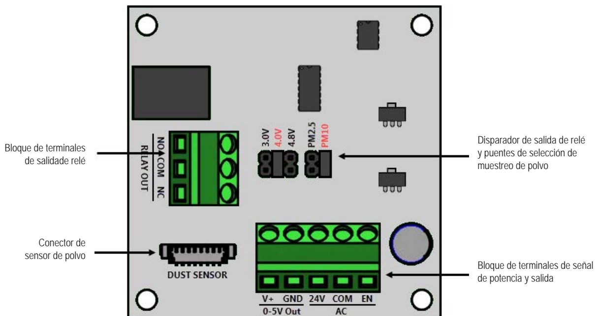
FIGURA 81 Placa de alarma del sensor de polvo 8612-064
