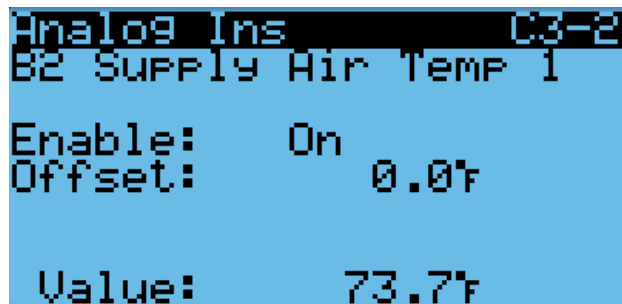
FIGURA 58 Sensor de temperatura del suministro de aire
