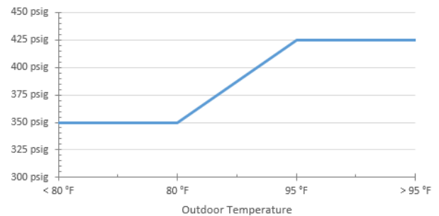
Descarga del ventilador del condensador / punto de ajuste de temperatura del líquido
