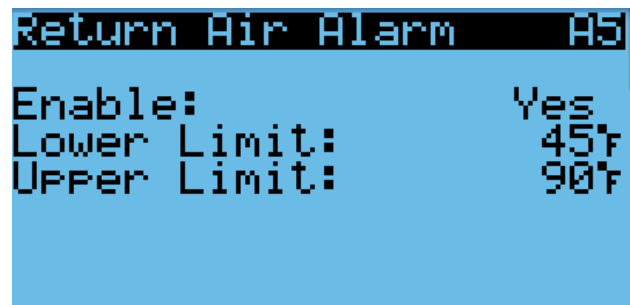
FIGURA 64 Modificación de los ajustes de la alarma del aire de retorno
