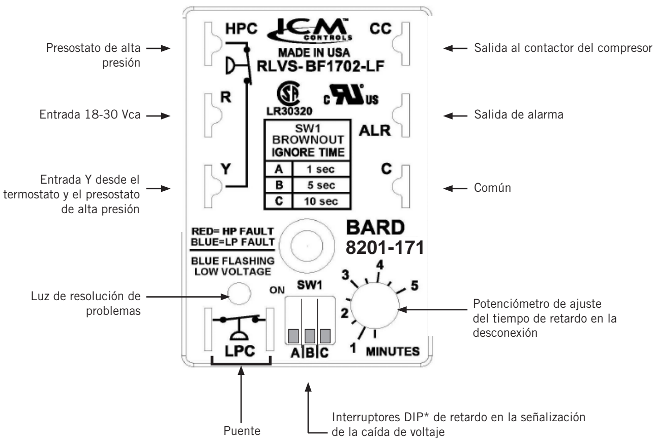
FIGURA 43 Módulo de control del compresor 8201-171
