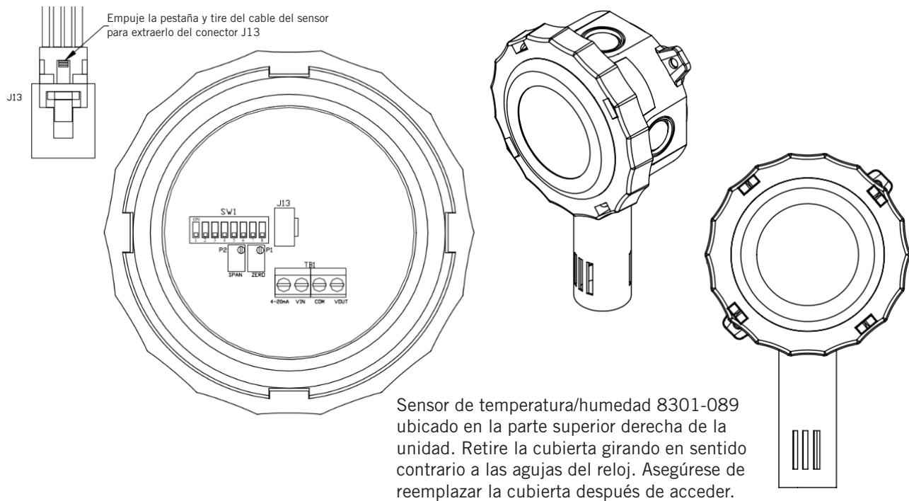
FIGURA 76 Conexiones eléctricas de sensores e interruptores DIP 8301-089
