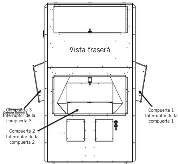
FIGURA 52 Las hojas de la compuerta
