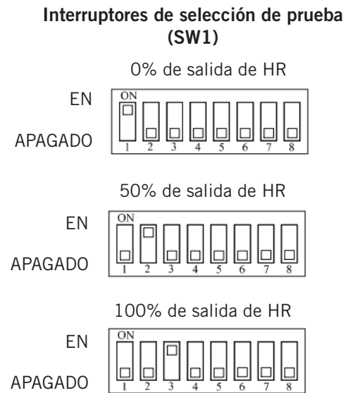
FIGURA 79 Configuración del conmutador/salida DIP 8301-089
