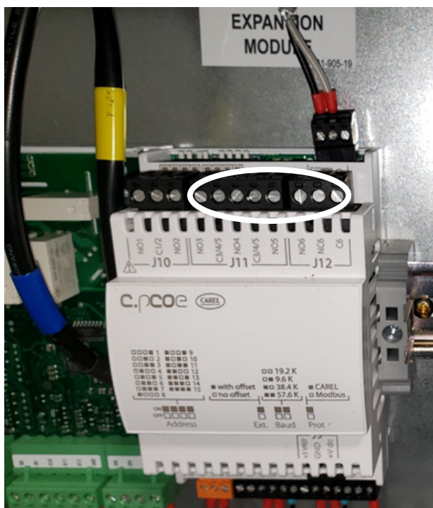
FIGURA 92 Ubicación del interruptor DIP
