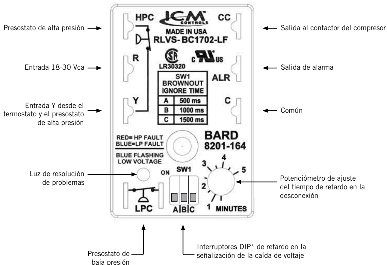
FIGURA 10 Módulo de control del compresor 8201-164
