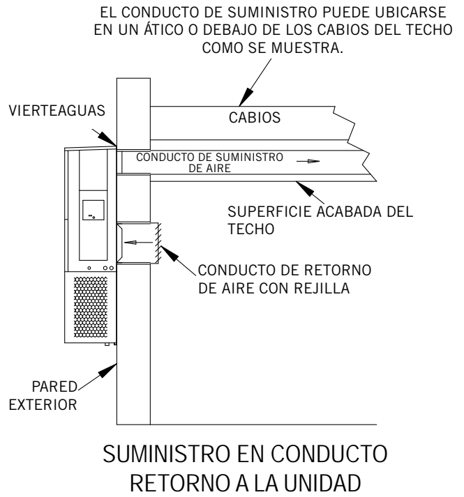
FIGURA 7 Instrucciones para el montaje en una pared común
