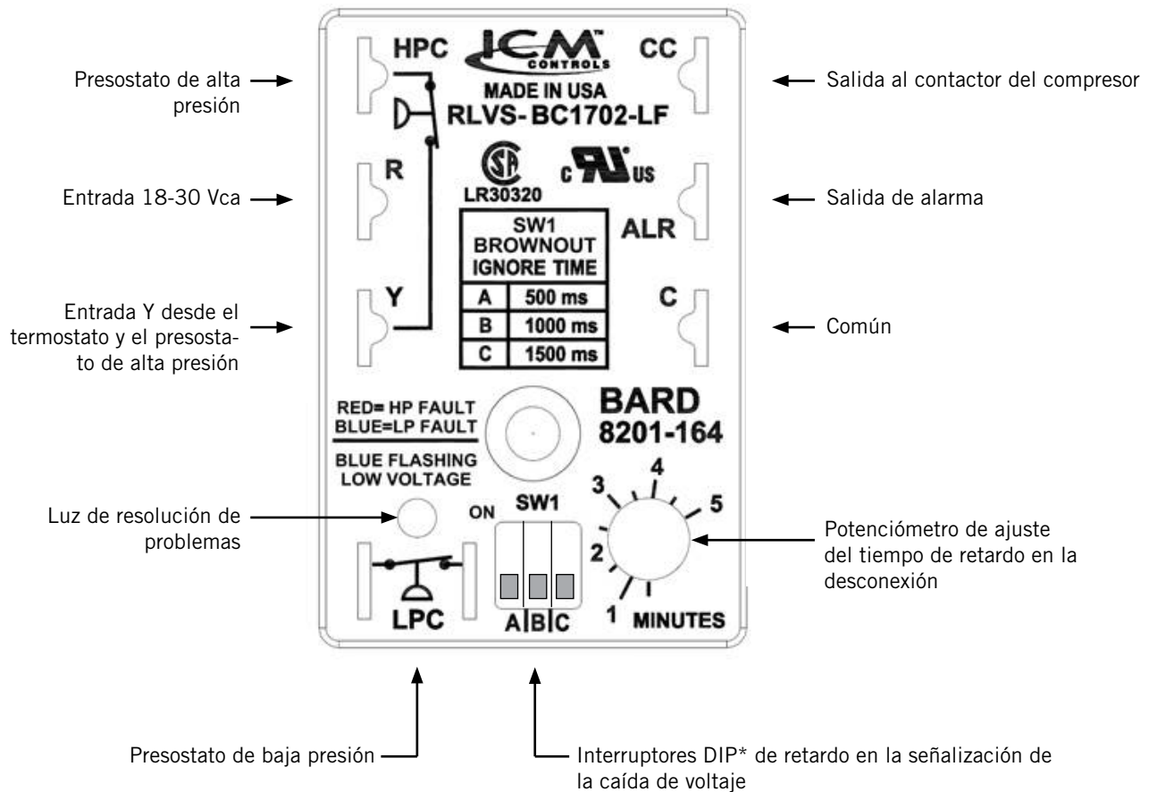
FIGURA 22 Módulo de control del compresor 8201-164
