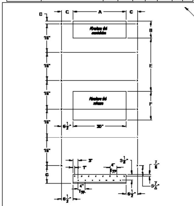
Vista de las aberturas en la pared y ubicación de los equipos
