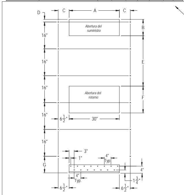
Vista de las aberturas en la pared y ubicación de los agujeros
