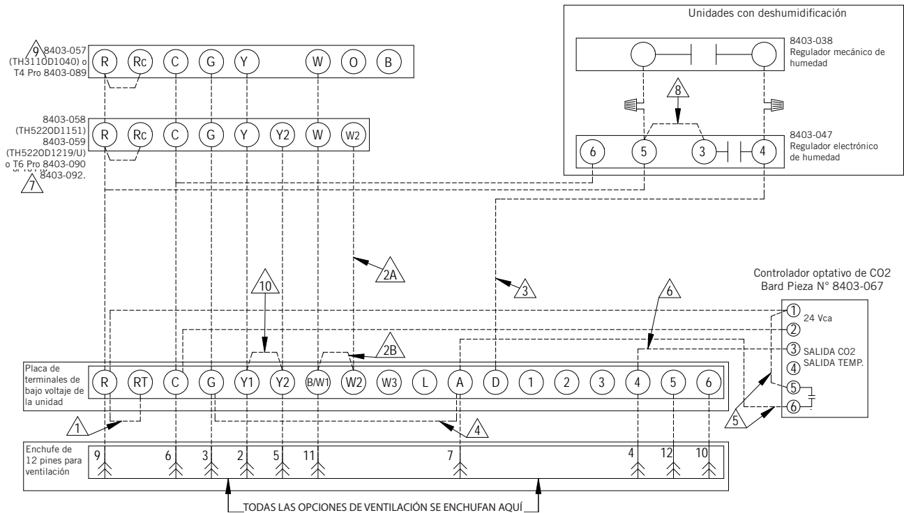
FIGURA 21 Conexiones del termostato no programable
