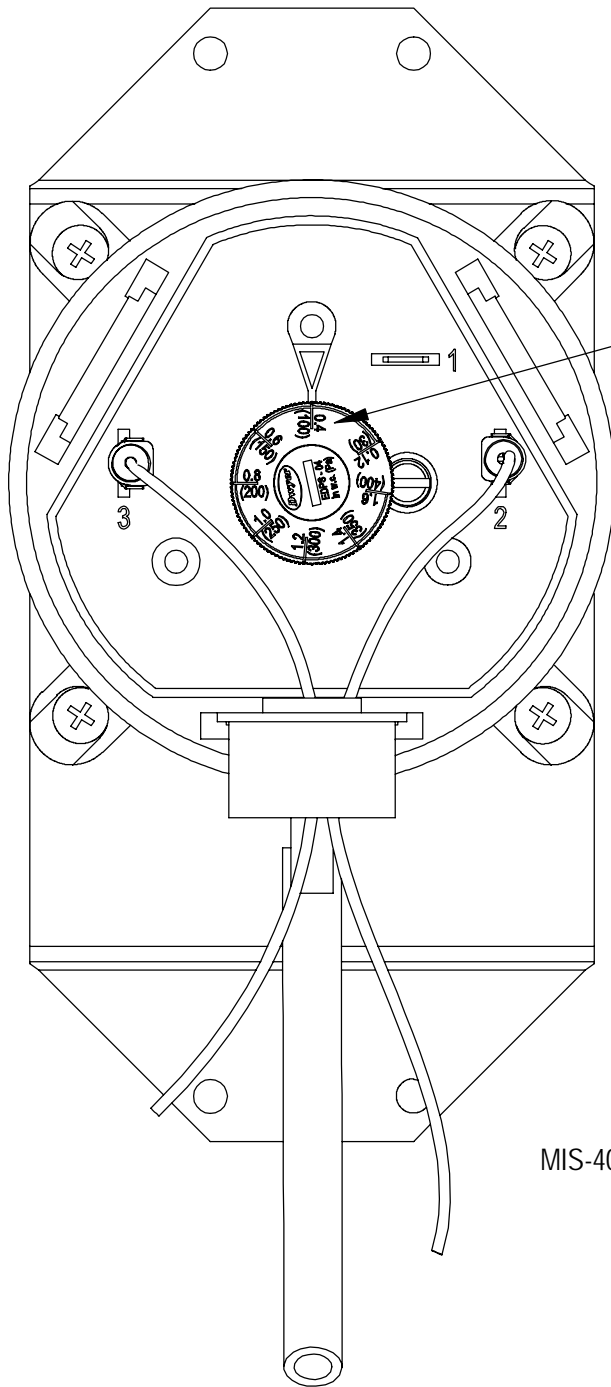
FIGURA 30 Ajuste del interruptor de filtro sucio
