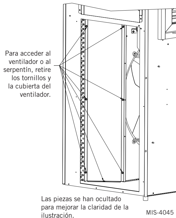
FIGURA 26 Desmontaje de la cubierta del ventilador
