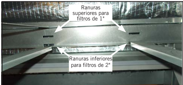
FIGURA 7 Vuelva a instalar los soportes de soporte del filtro en las ranuras inferiores
