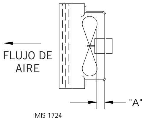
FIGURA 25 Regulación de las paletas del ventilador
