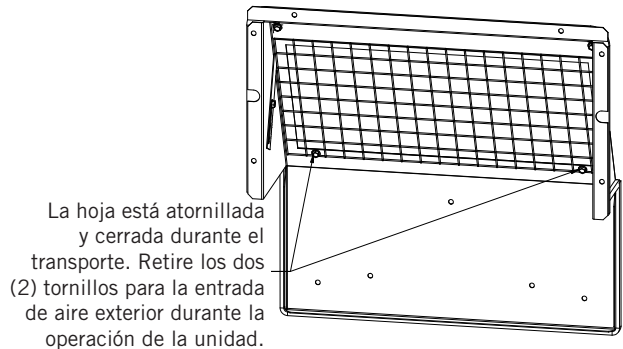
FIGURA 11 Compuerta reguladora de aire fresco
