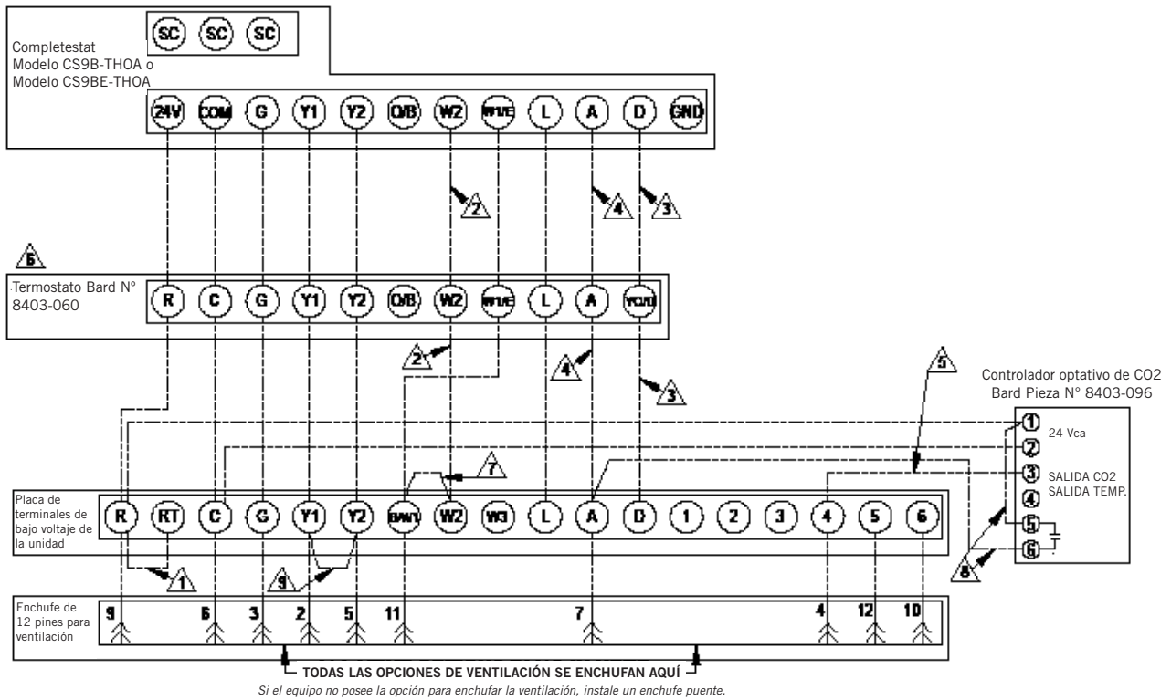
FIGURA 20 Conexiones del termostato programable
