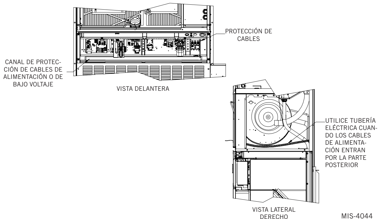
FIGURA 19 Conexiones de voltaje de red
