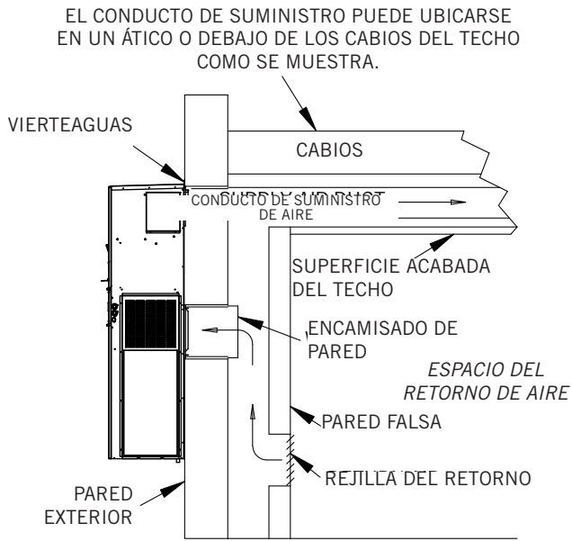
INSTALACIÓN EN PARED FALSA
