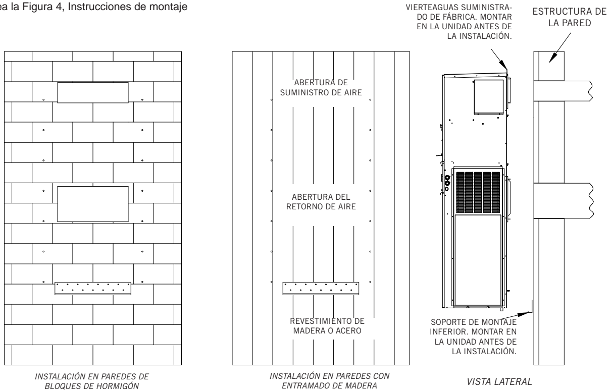
FIGURA 16 Instrucciones para montaje en pared
