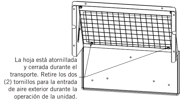
FIGURA 11 Compuerta reguladora de aire fresco
