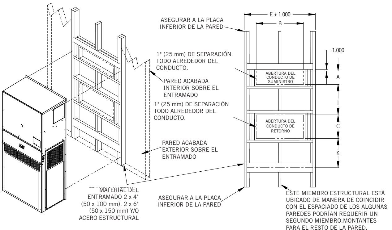
FIGURA 17 Instrucciones para montaje en pared
