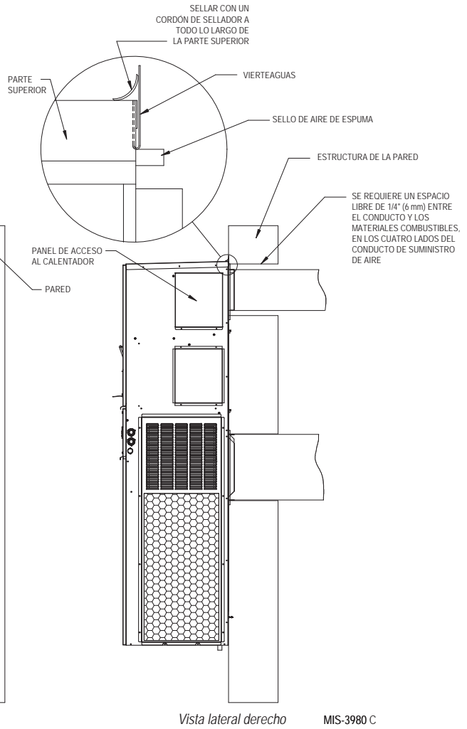
FIGURA 14 Instrucciones de montaje
