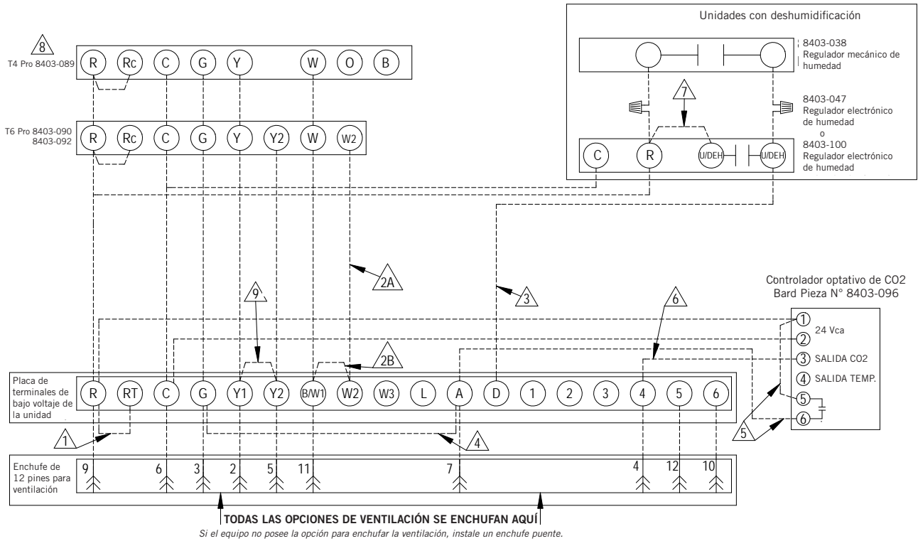
FIGURA 21 Conexiones del termostato no programable
