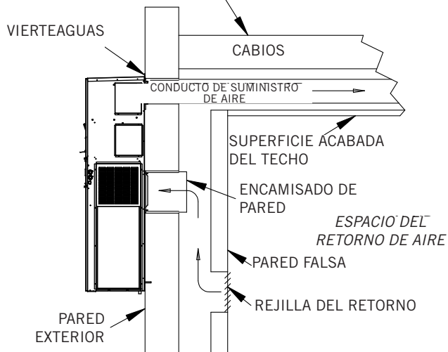
INSTALACIÓN EN PARED FALSA
