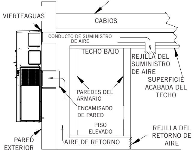
INSTALACIÓN EN ARMARIO
