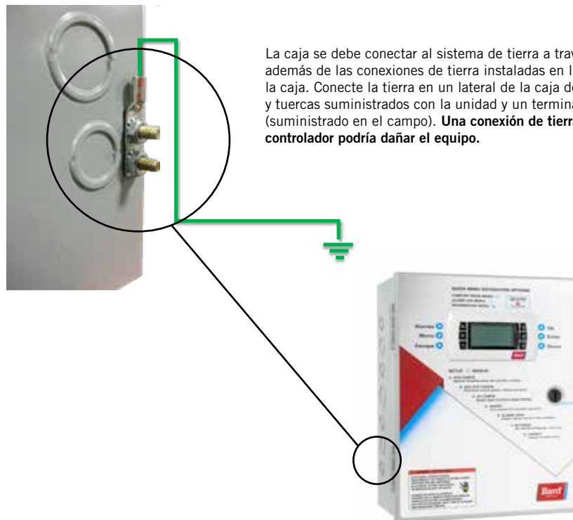
FIGURA 27 Pernos de conexión a tierra del controlador
