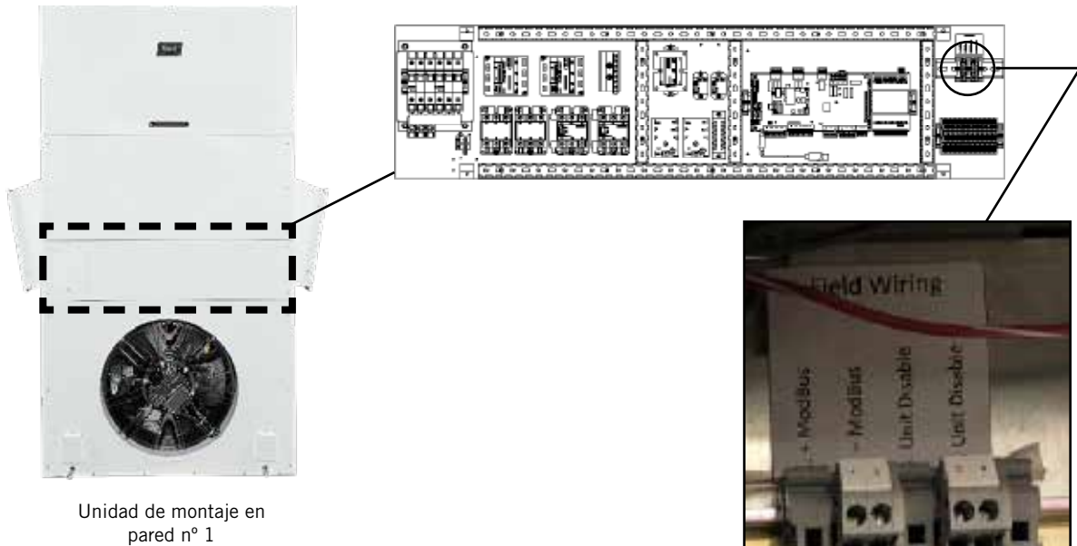
FIGURA 24 Cableado de comunicación: Terminación en la primera unidad de montaje en pared
