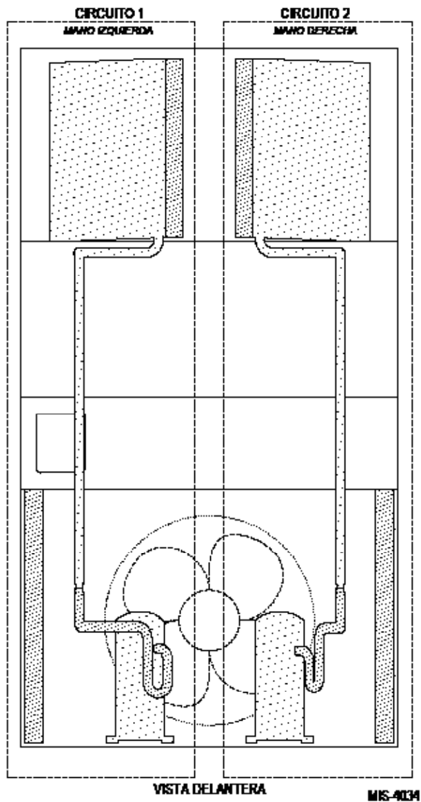
Circuitos de enfriamiento de la unidad MEGA-TEC
