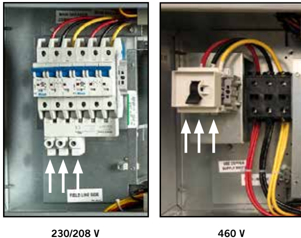
FIGURA 10 Puntos de conexión de la alimentación en Vca
