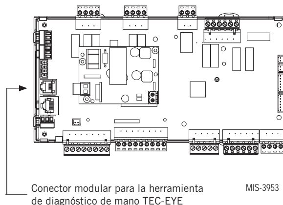
FIGURA 29 Conexión de TEC-EYE con la unidad de control
