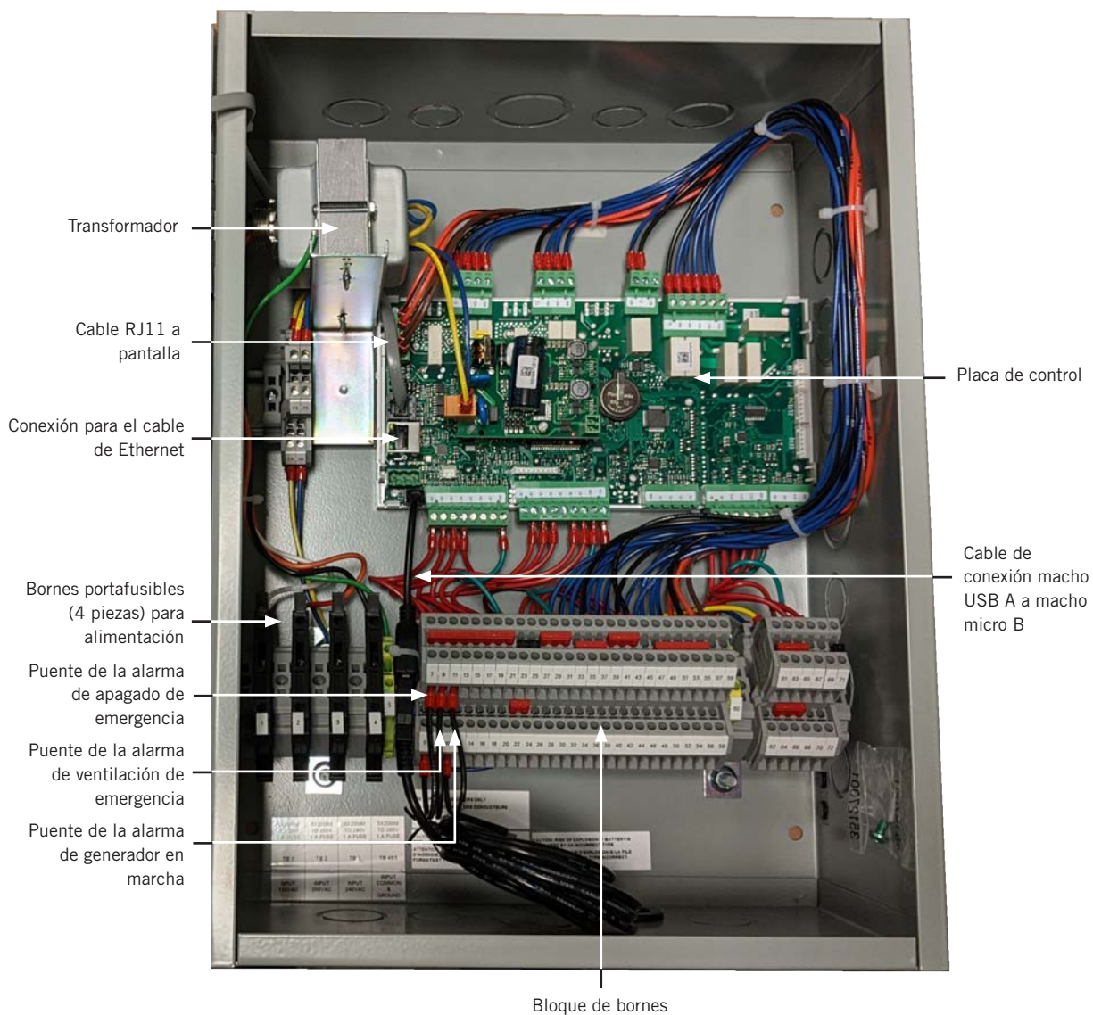
FIGURA 14 Ubicación habitual de los componentes del LC6000-200
