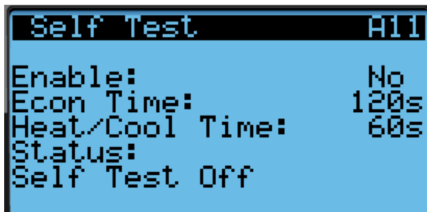
FIGURA 32 Ejecución de una prueba de funcionamiento
