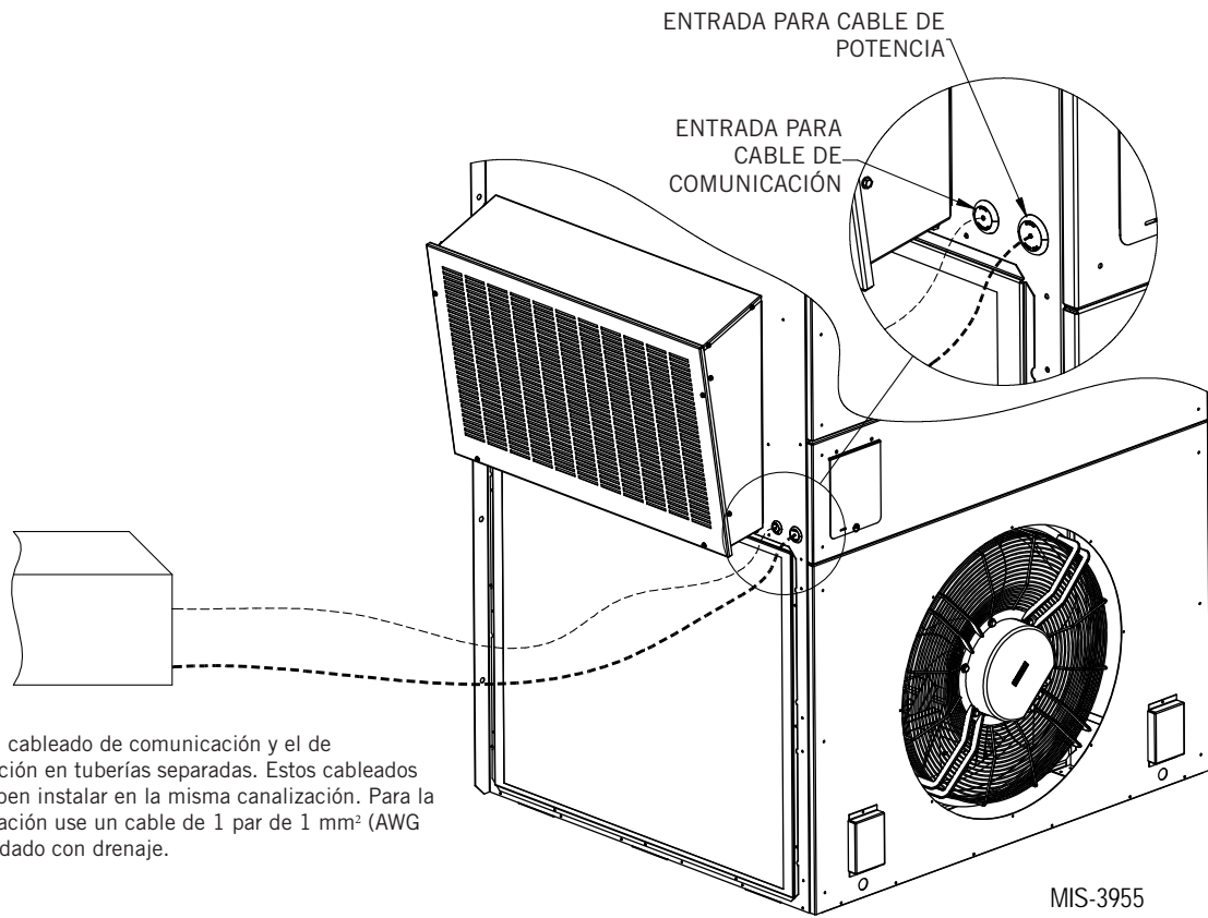
FIGURA 12 Entradas posteriores para cables de comunicación y potencia (opcionales)
