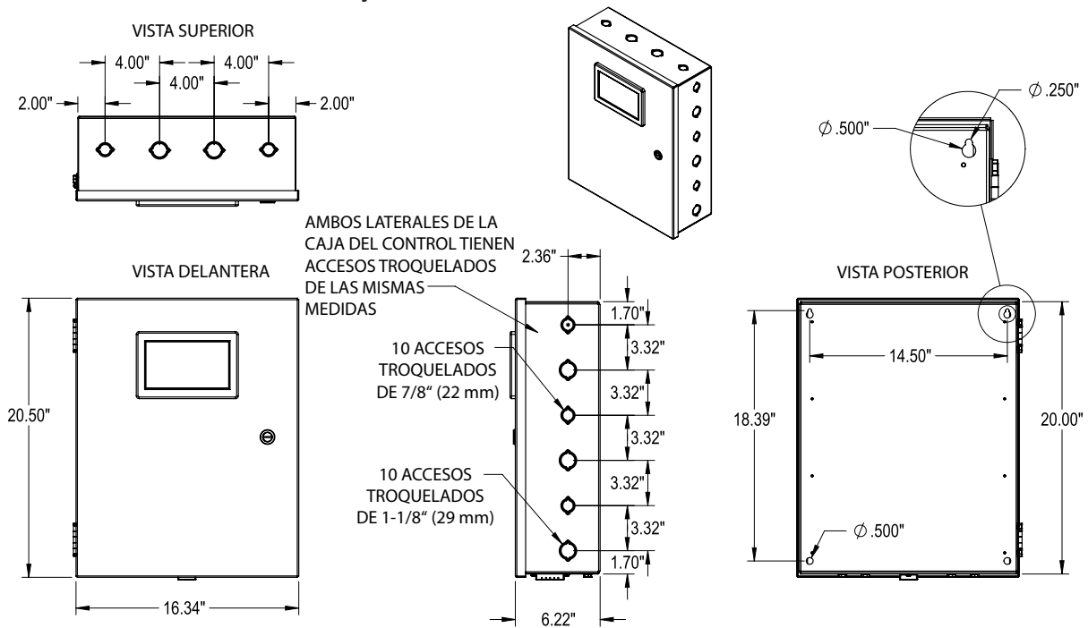
FIGURA 2 Dibujo dimensional del controlador MC5000
