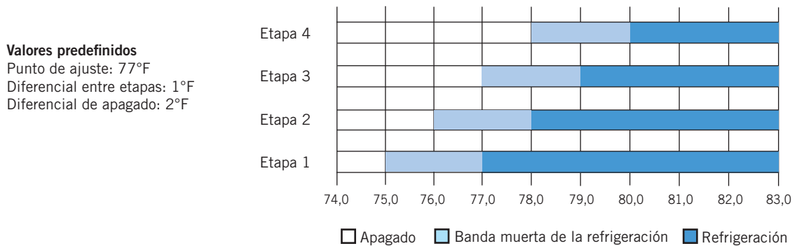
FIGURA 11 Refrigeración con seis unidades de una etapa (c/economizadores) usando la opción de hermanamiento triple
